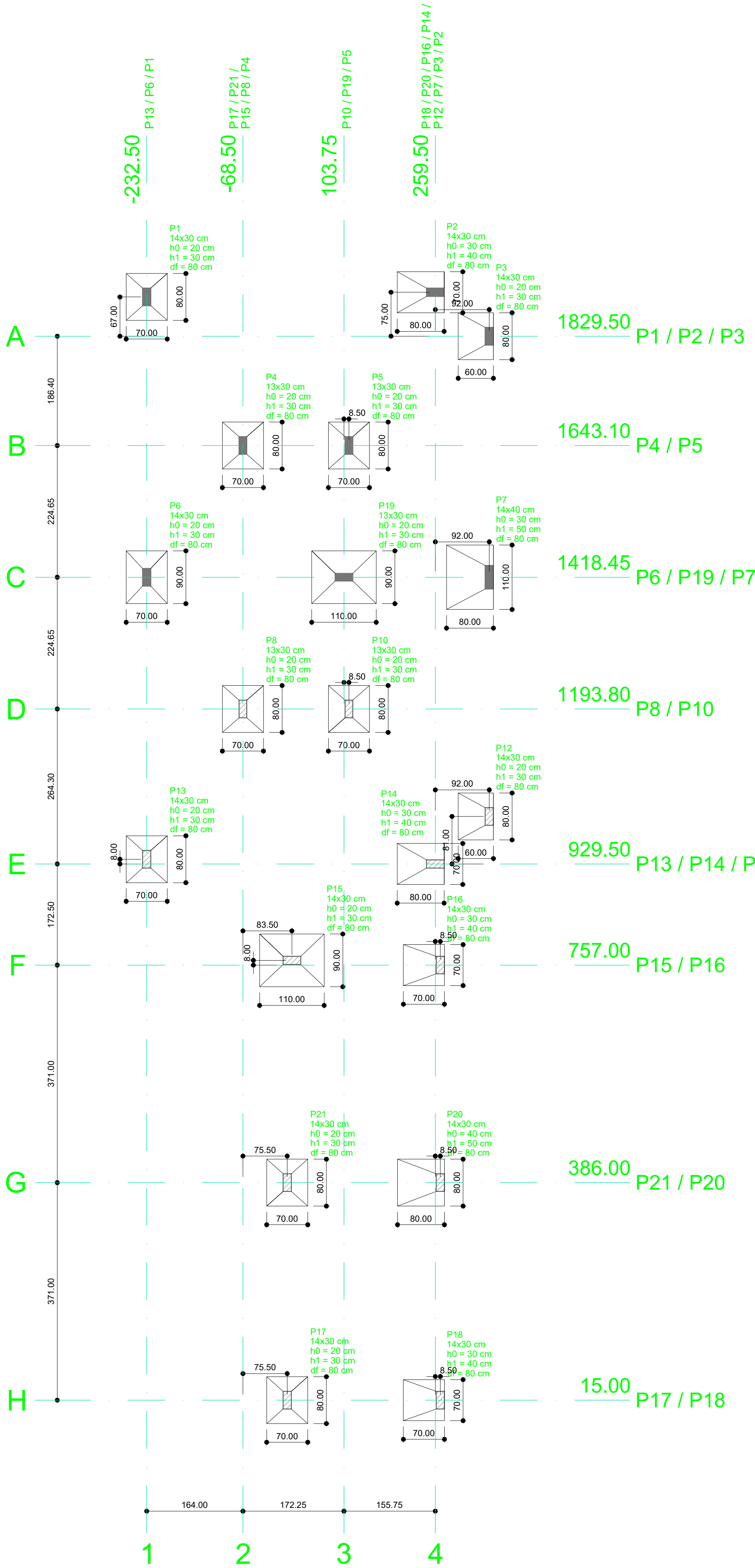
Planta de Locação das Sapatas escala 1:50
