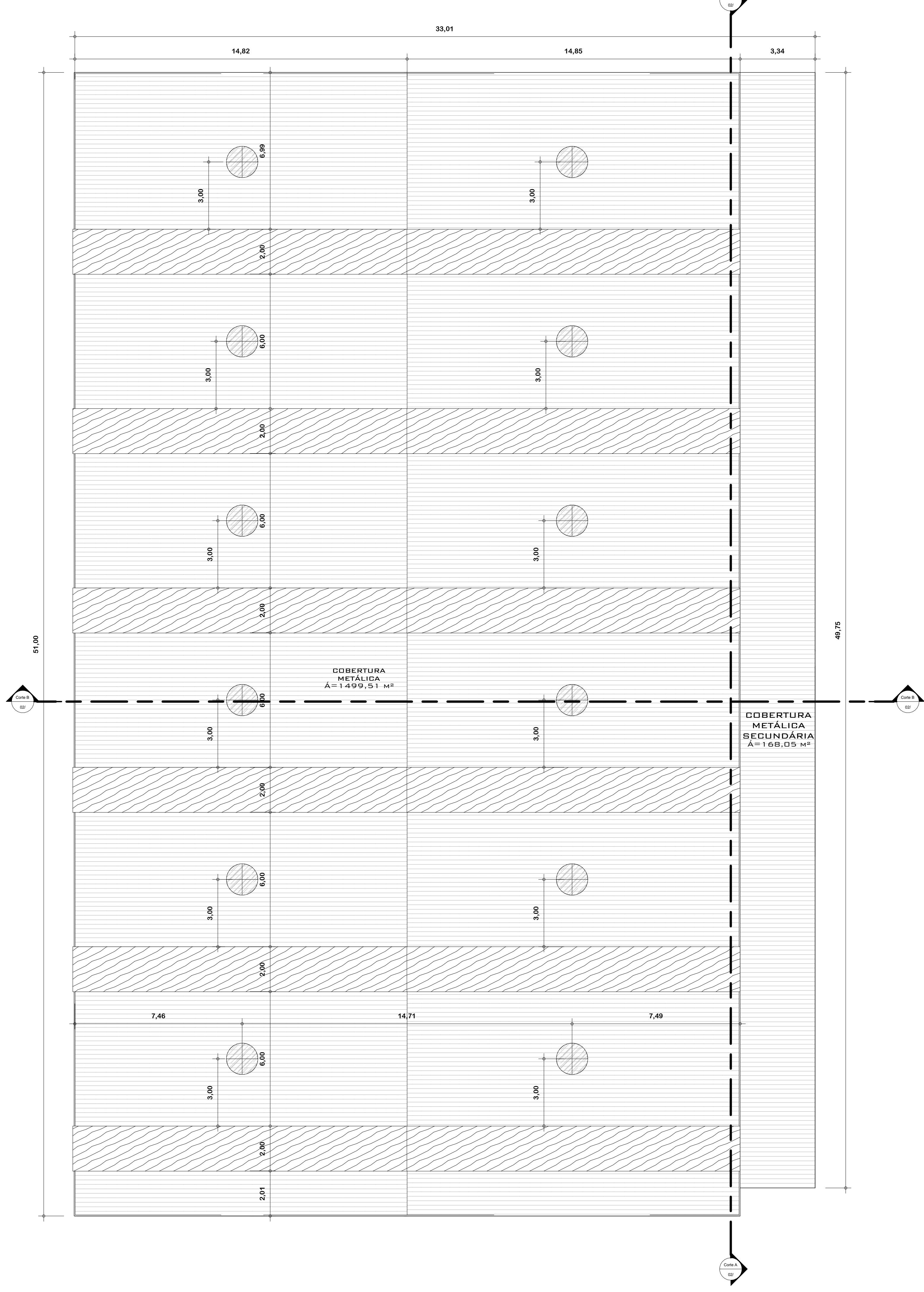
2 COBERTURA 1 : 100
