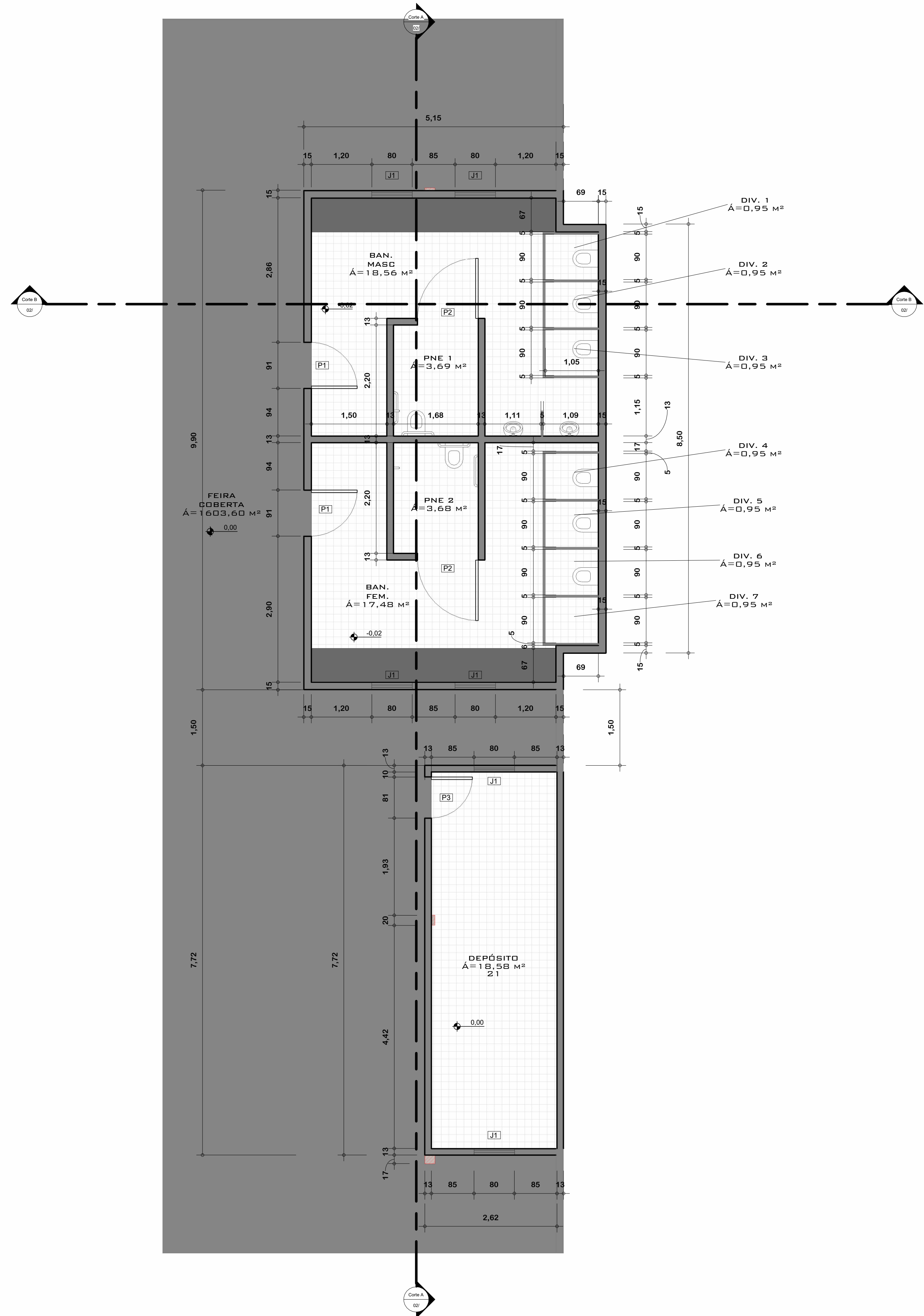
3 DETALHE 1 1 : 50
