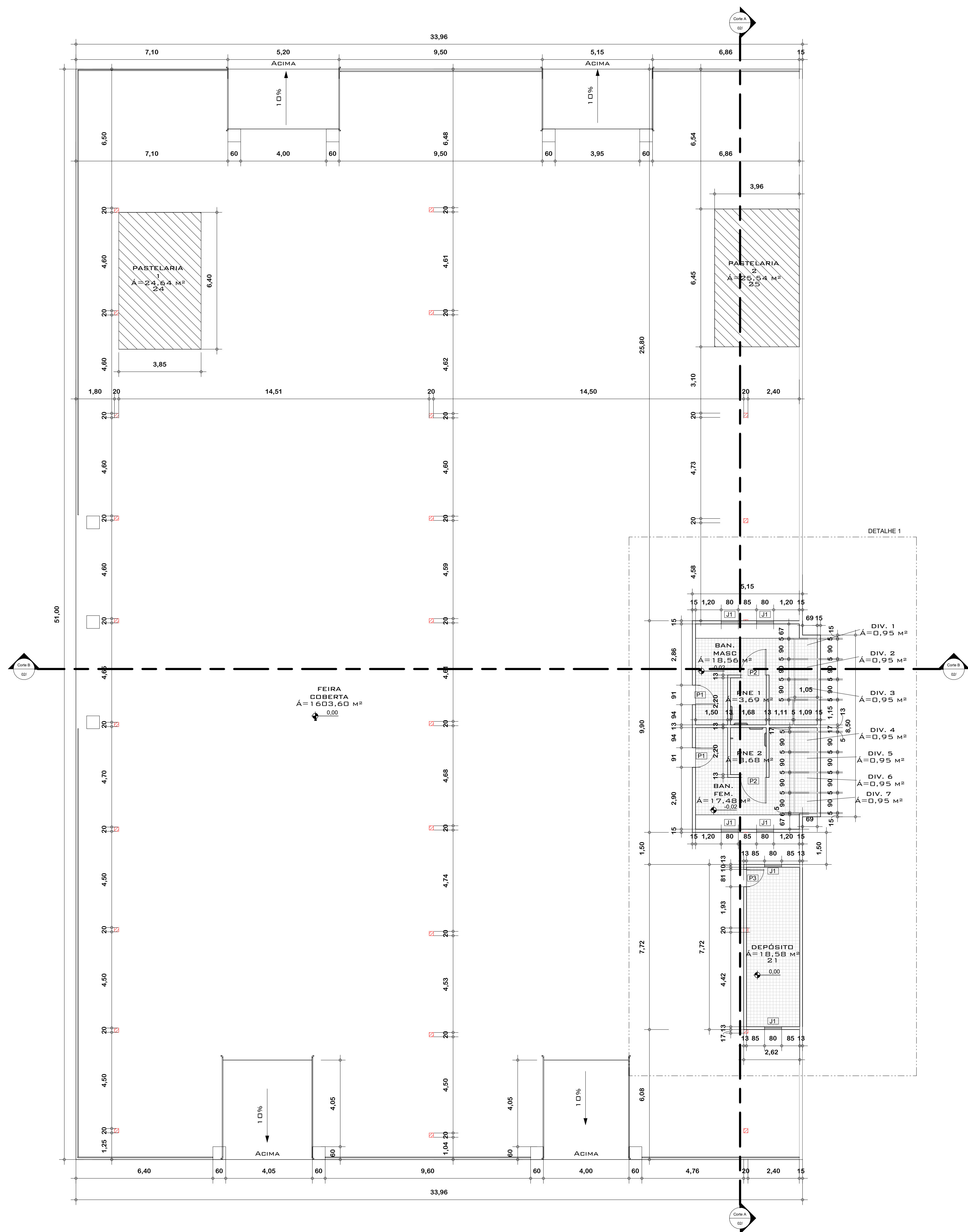
1 PAVIMENTO TÉRREO 1 : 100
