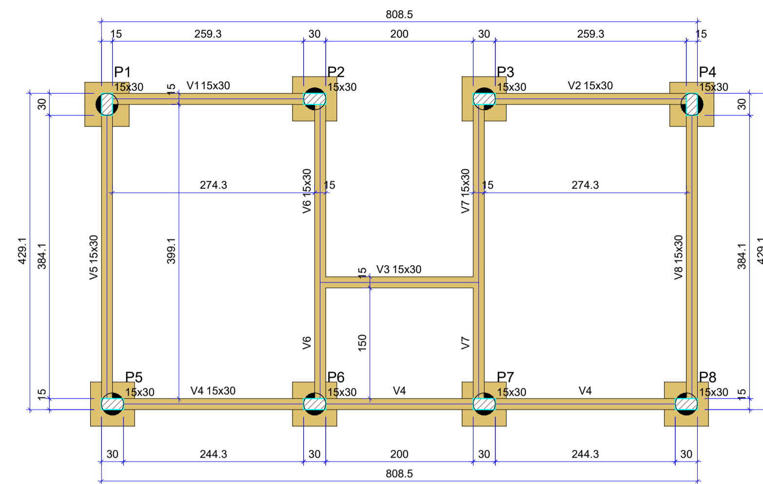
Forma do pavimento BALDRAME escala 1:50
