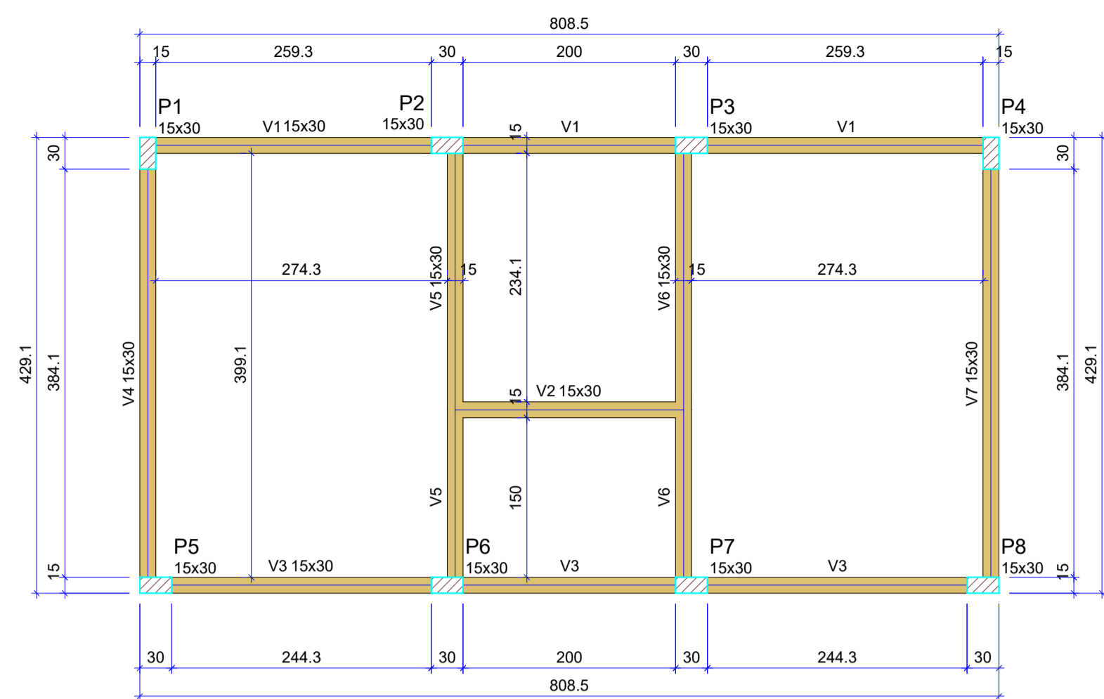
Forma do pavimento TERREO escala 1:50
