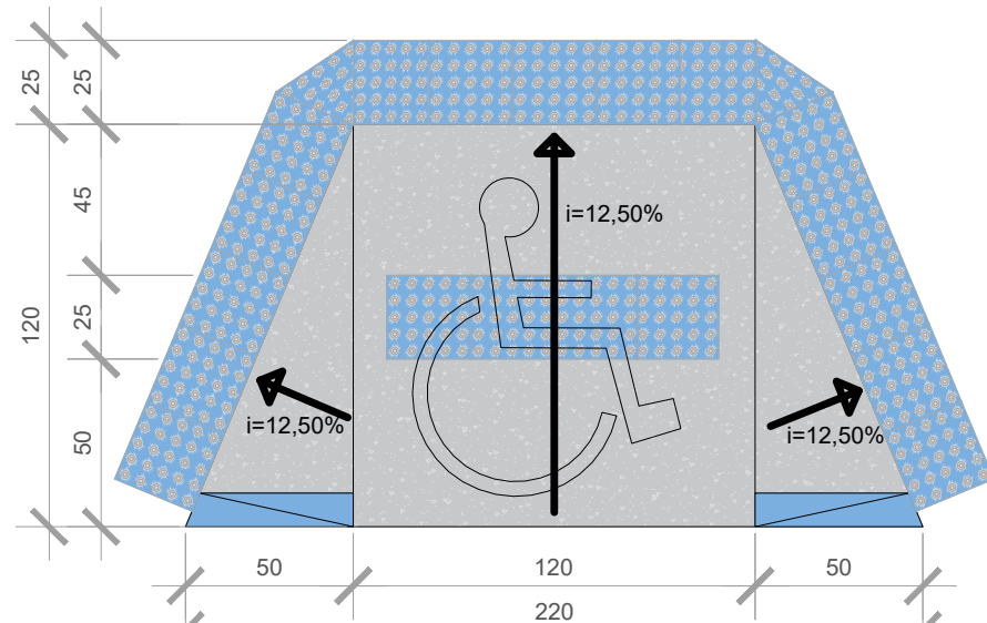
Det. Rampa de Acessibilidade esc.: 1:25
