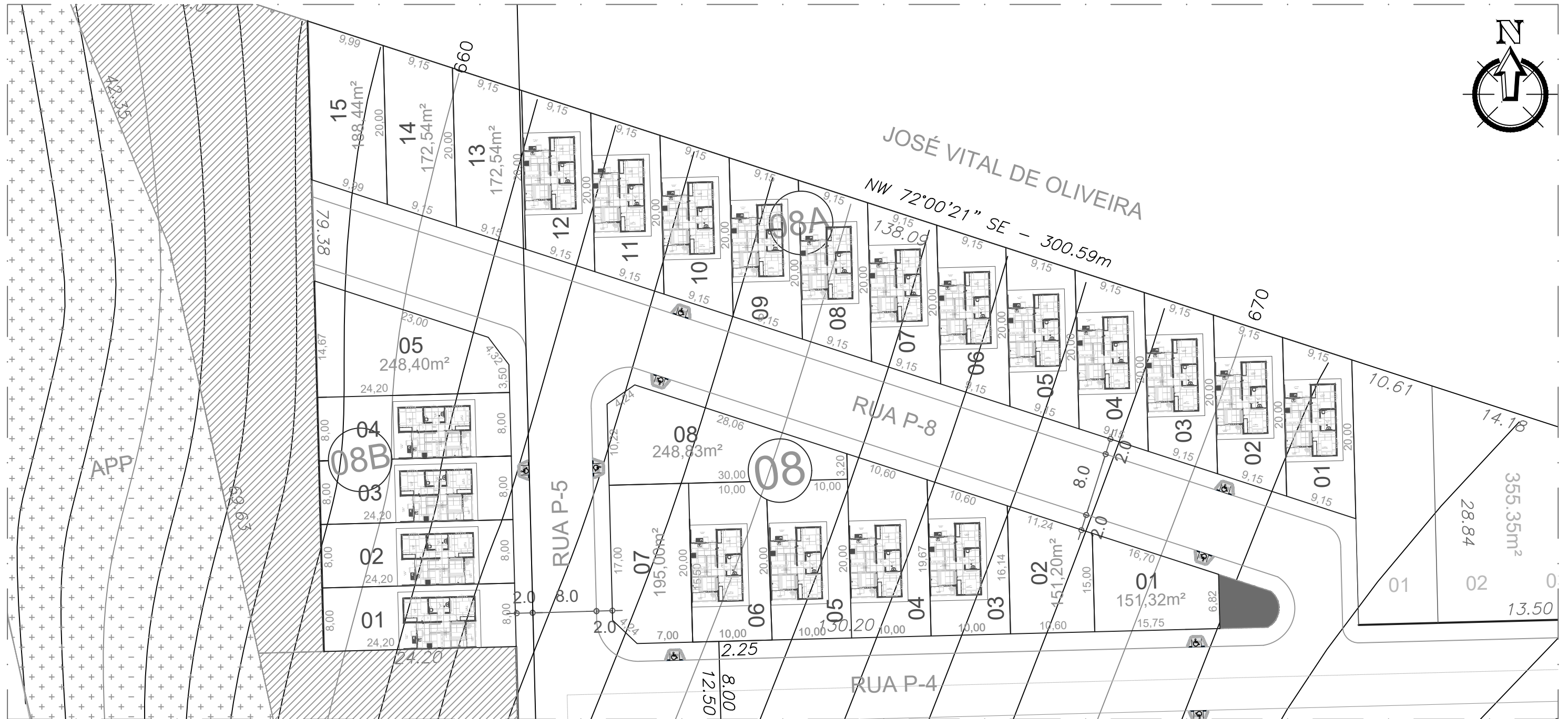
Projeto de Acessibilidade de Calçada esc.: 1:500
