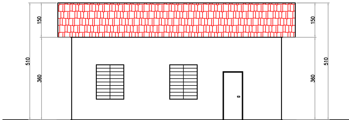
VISTA 2 ESC.: 1:100
