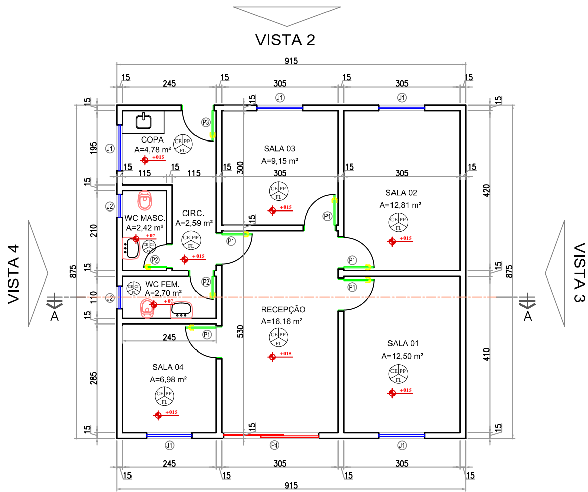
PLANTA BAIXA ESC.: 1:100
