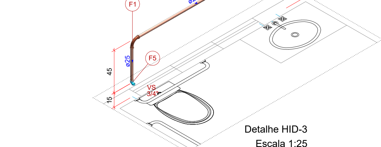
Detalhe HID-3 Escala 1:25
