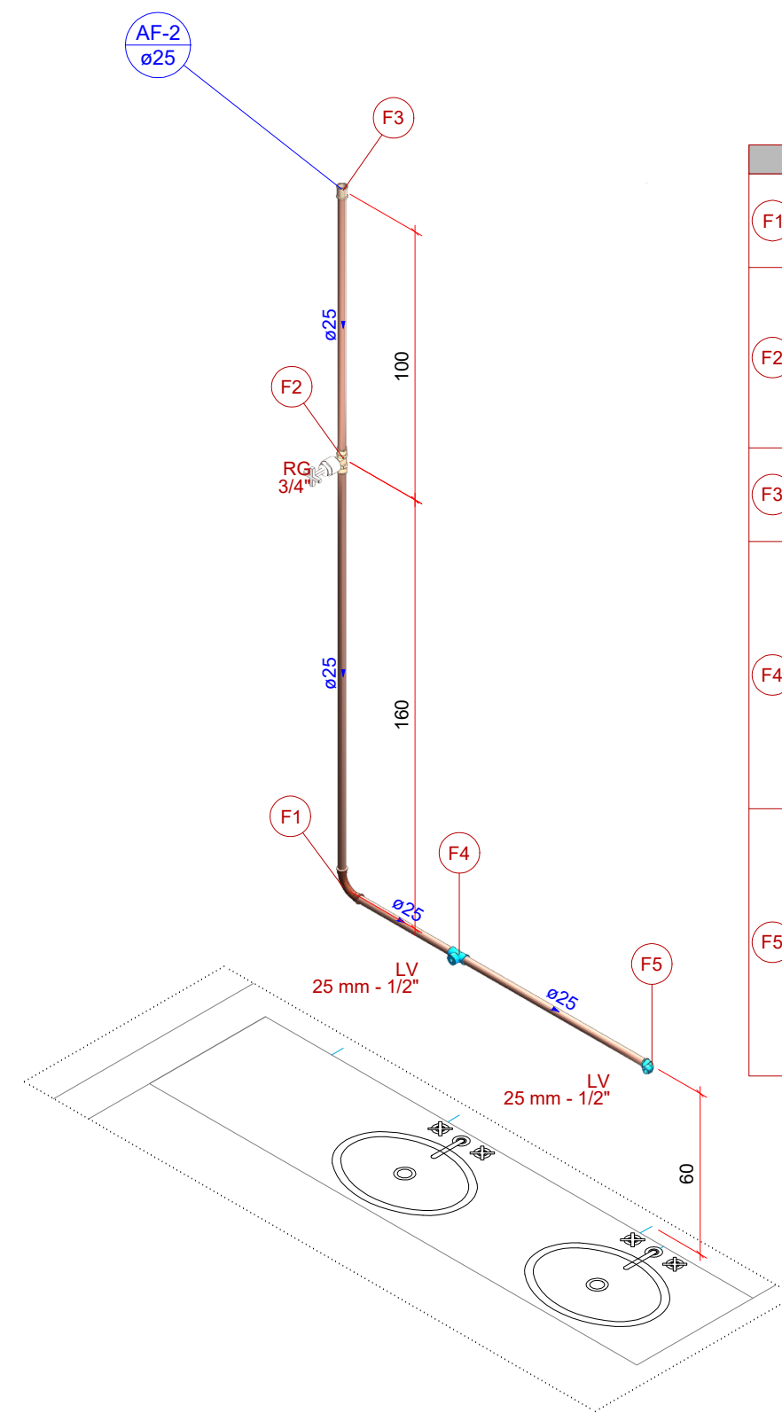
Detalhe HID-2 Escala 1:25
