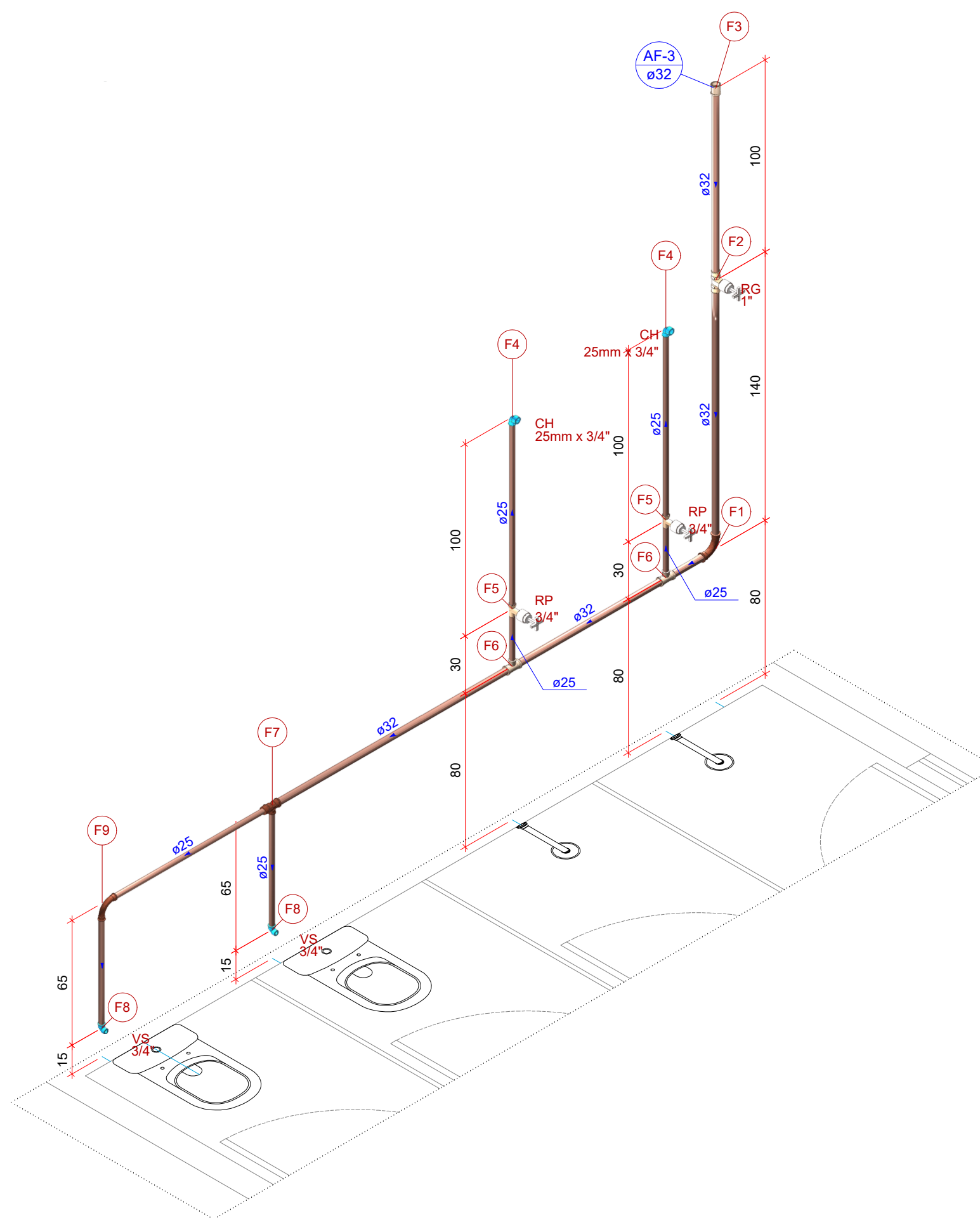
Detalhe HID-4 Escala 1:25
