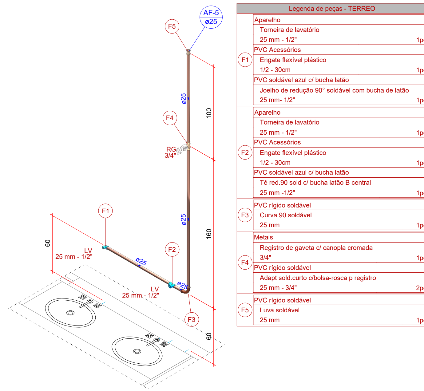
Detalhe HID-6 Escala 1:25
