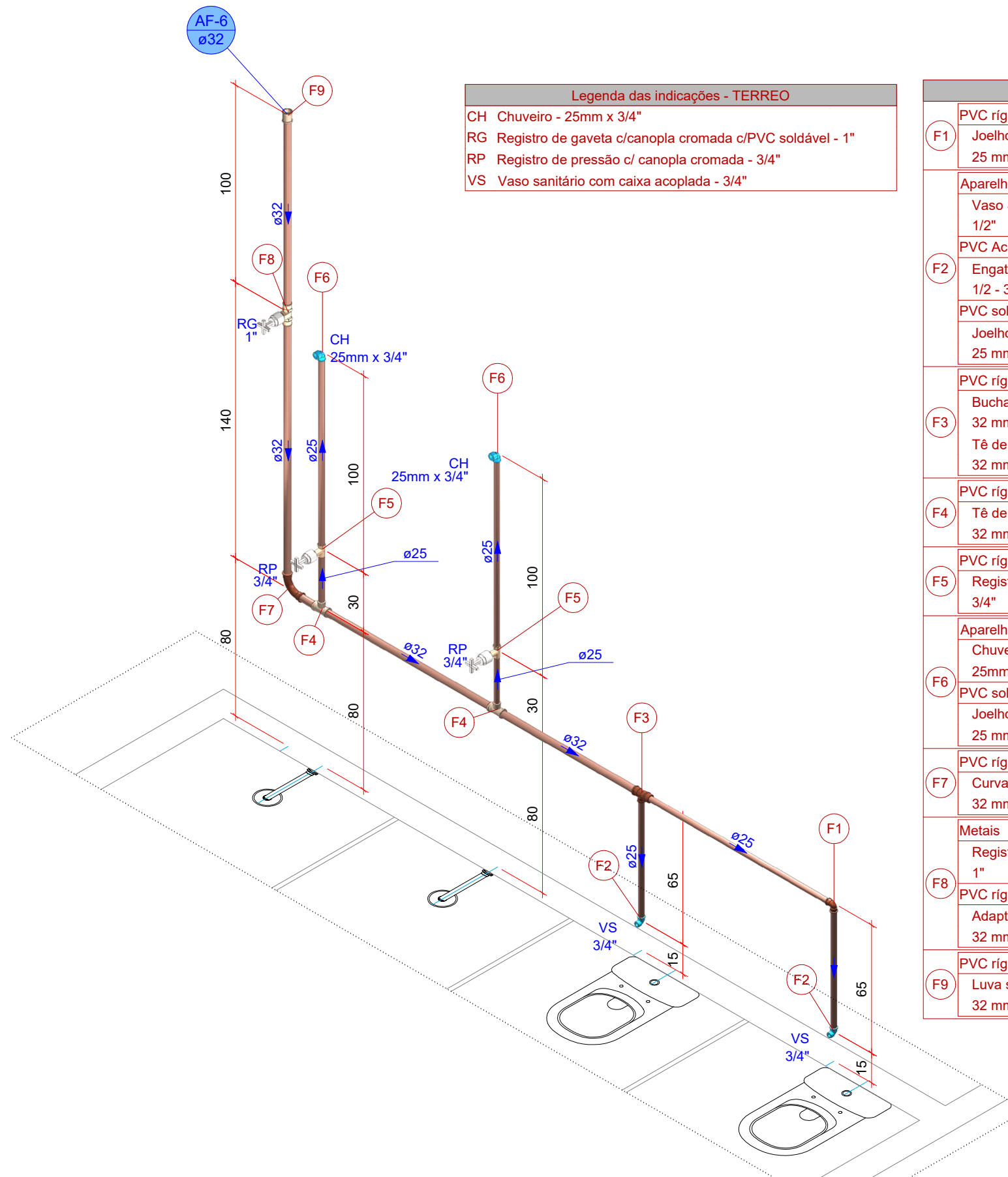
Detalhe HID-1 Escala 1:25
