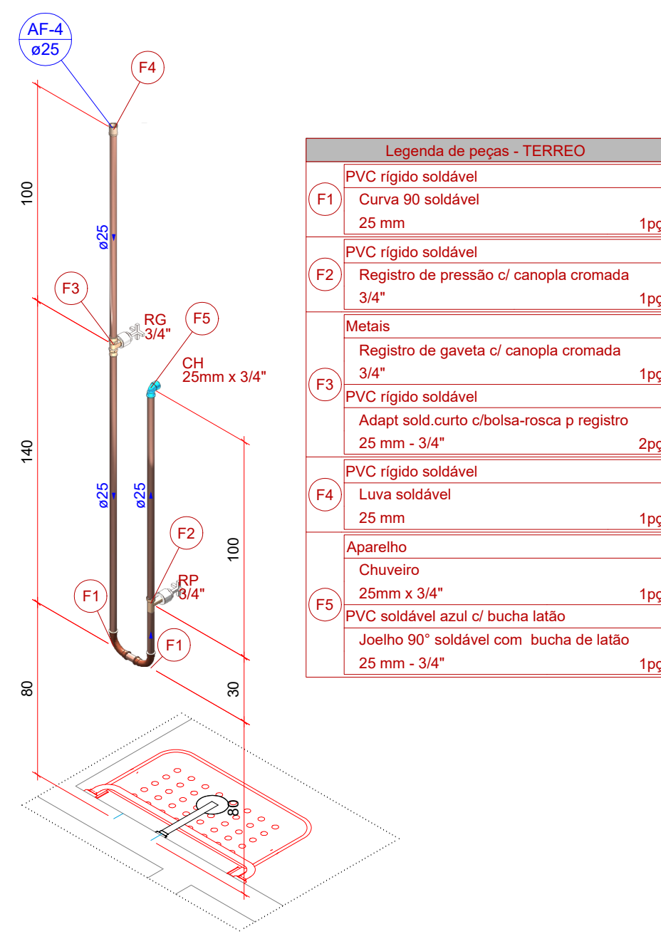
Detalhe HID-5 Escala 1:25
