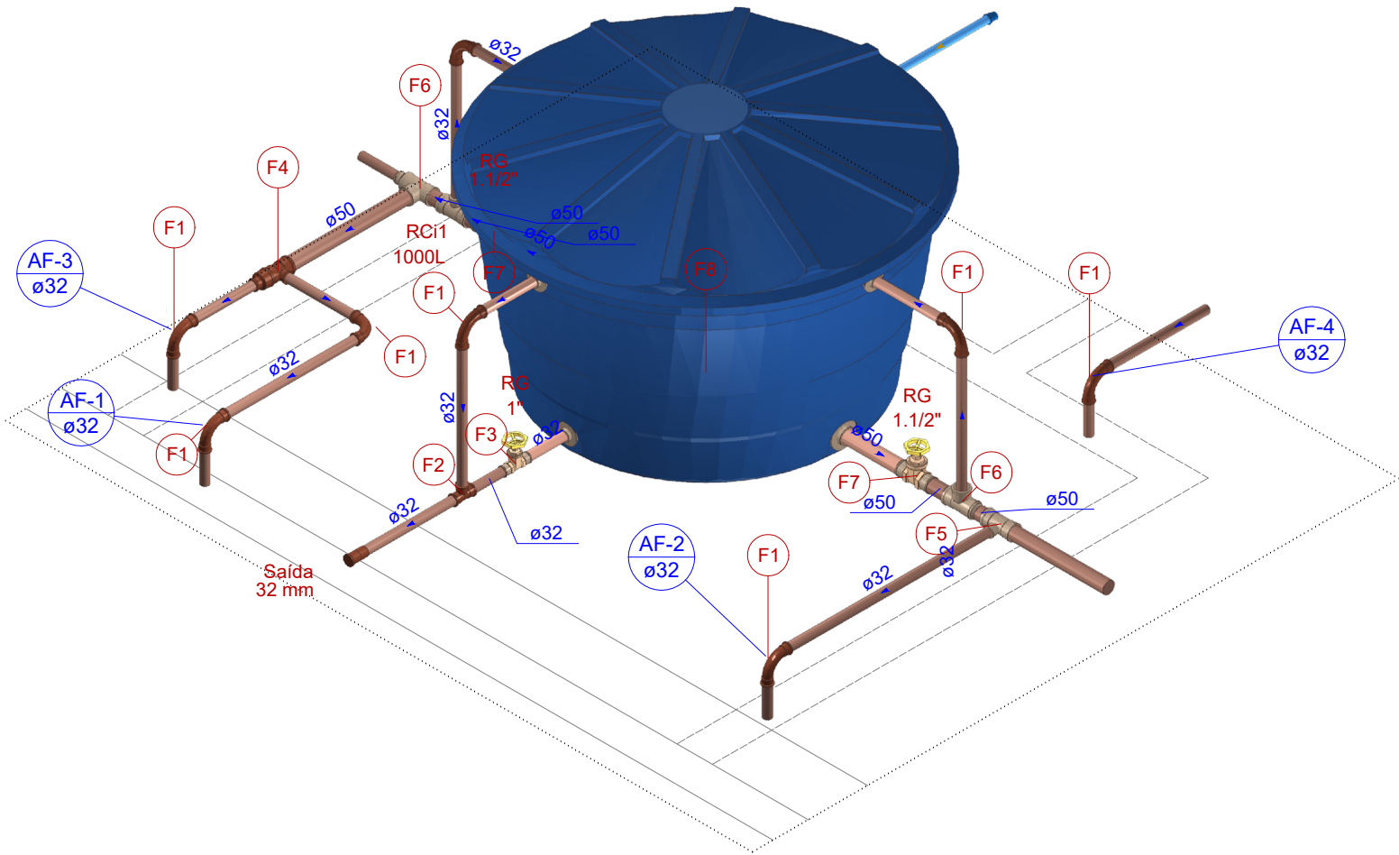
Detalhe HID-7 Escala 1:25
