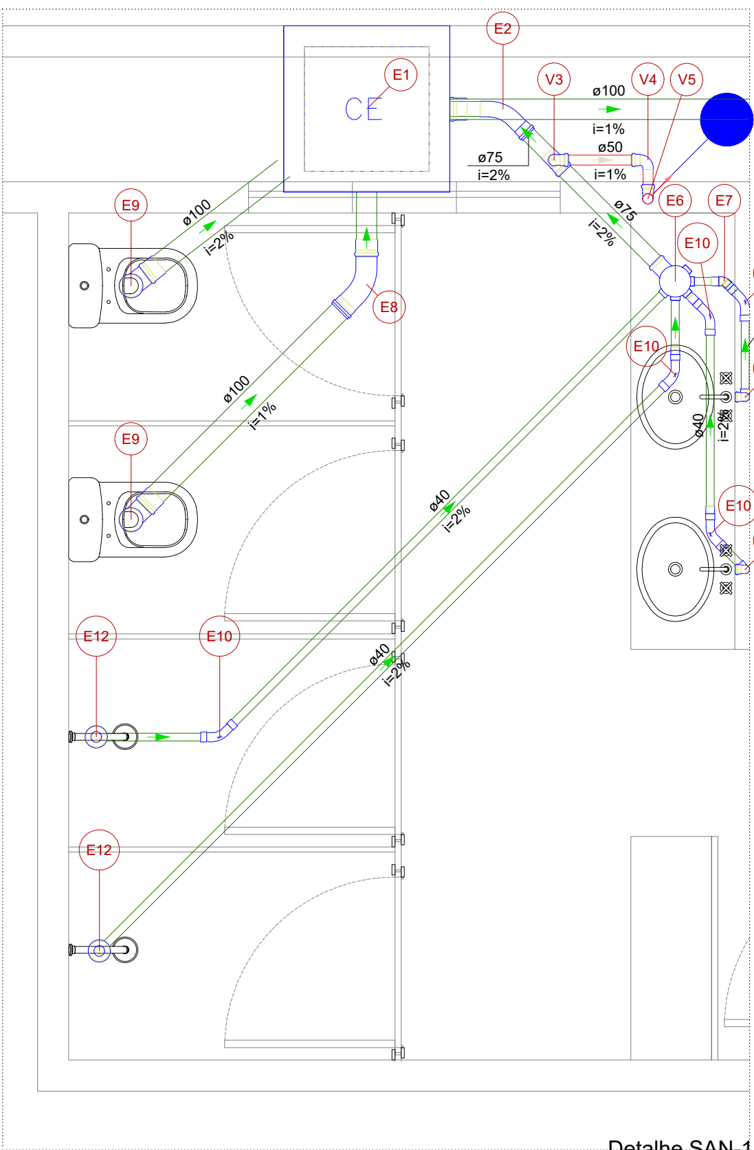
Detalhe SAN-1 Escala 1:25
