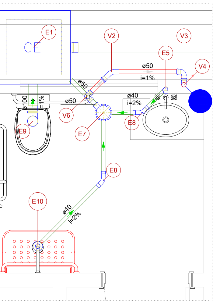
Detalhe SAN-2 Escala 1:25
