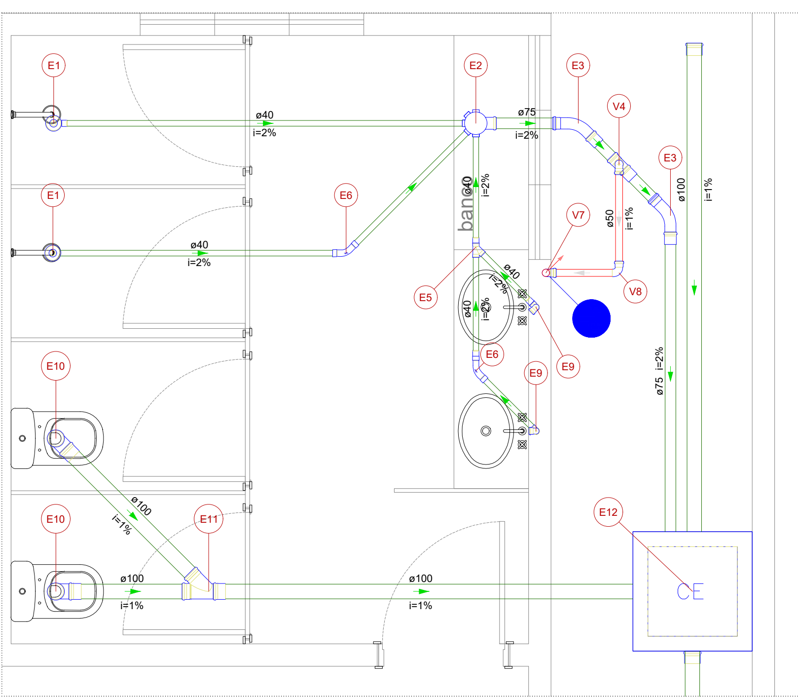
Detalhe SAN-4 Escala 1:25
