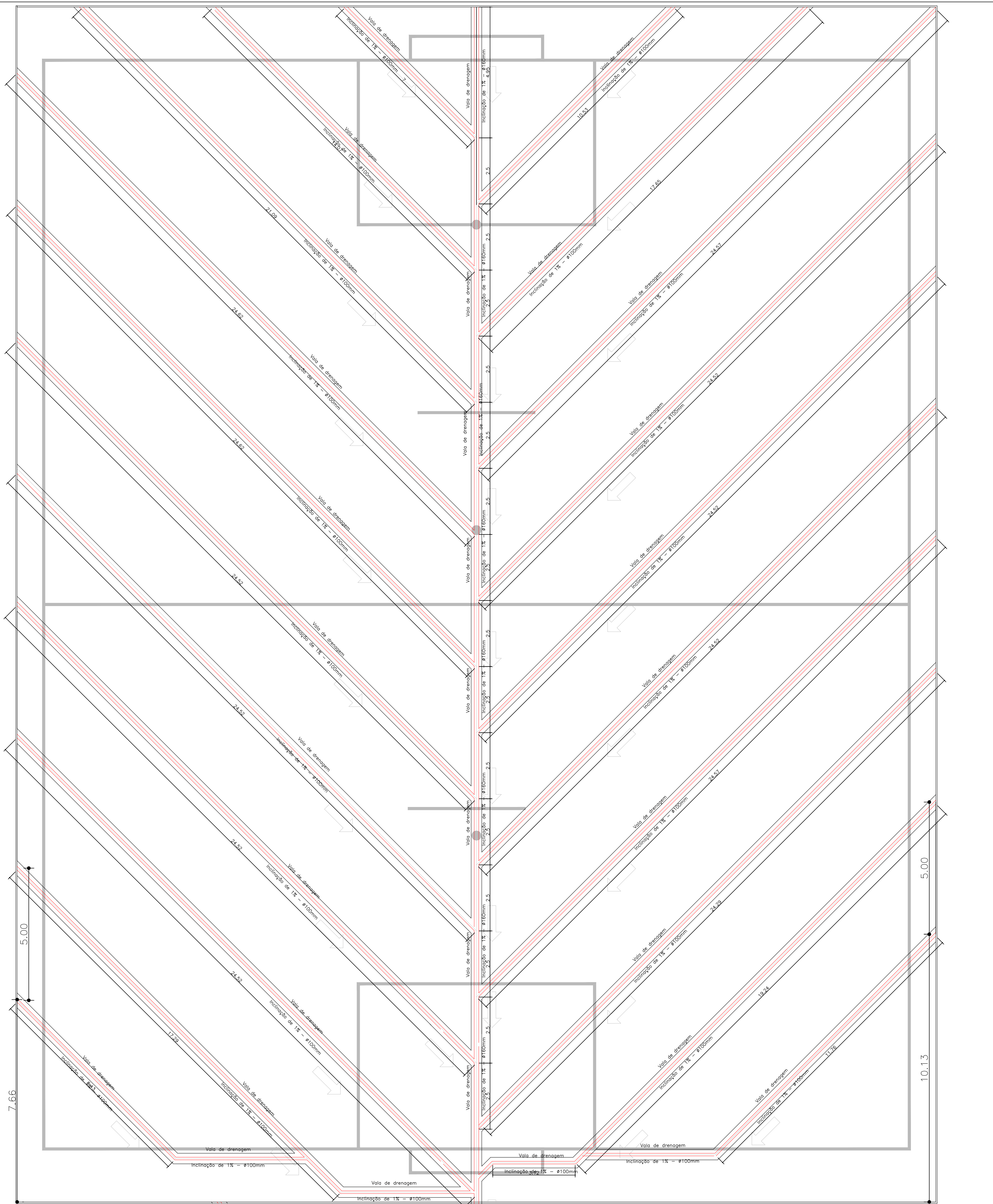
PLANTA – SISTEMA DE DRENAGEM ESC. 1:75
