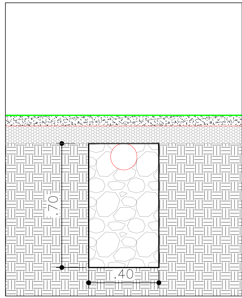
INICIO DA DRENAGEM SEM ESCALA
