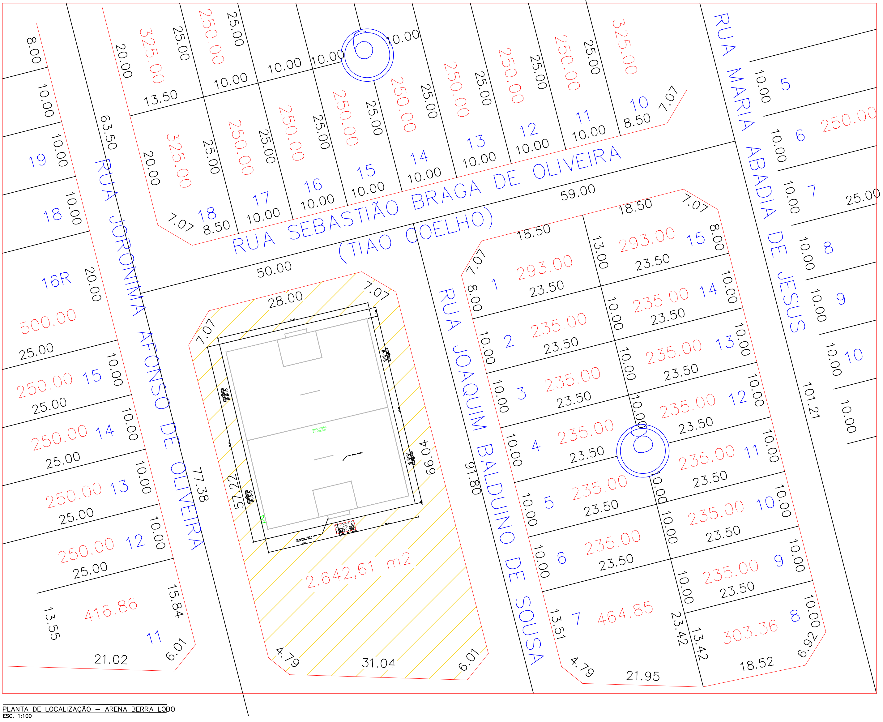
PLANTA DE LOCALIZAÇÃO – ARENA BERRA LOBO ESC. 1:100
