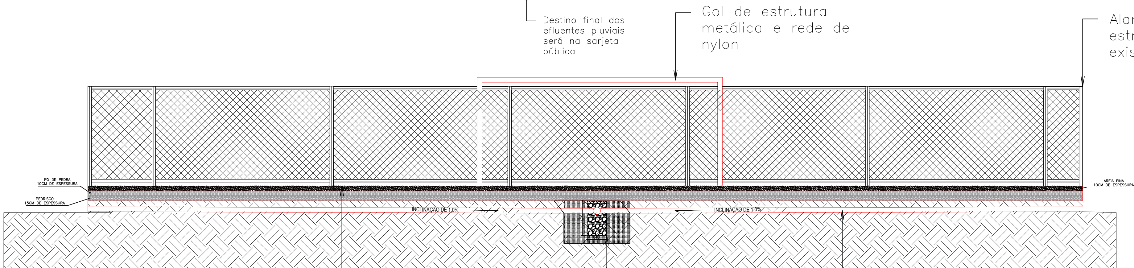
CORTE AA – CAMPO SOCIETY ESC. 1:100
