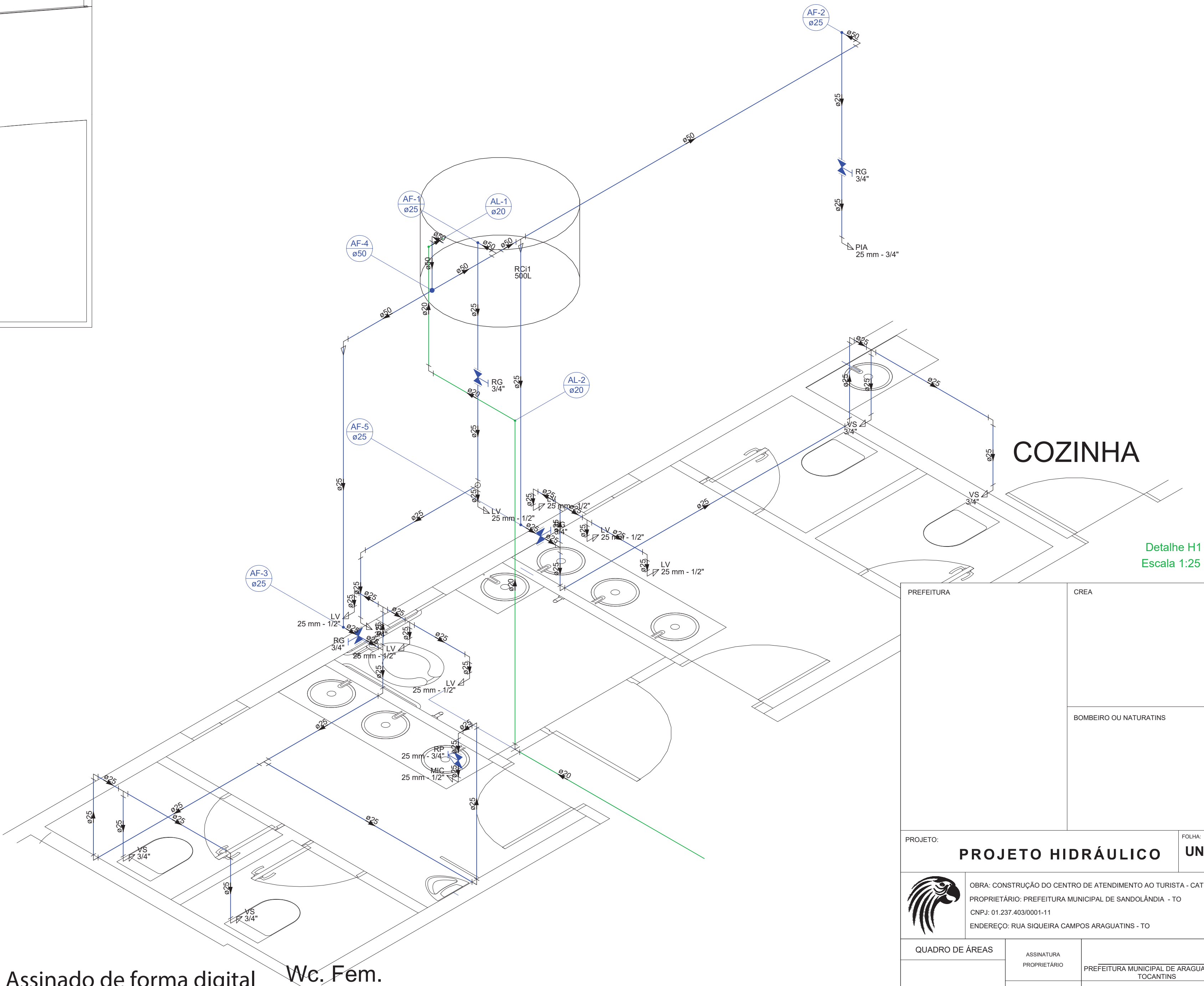
Detalhe H2 Escala 1:25
