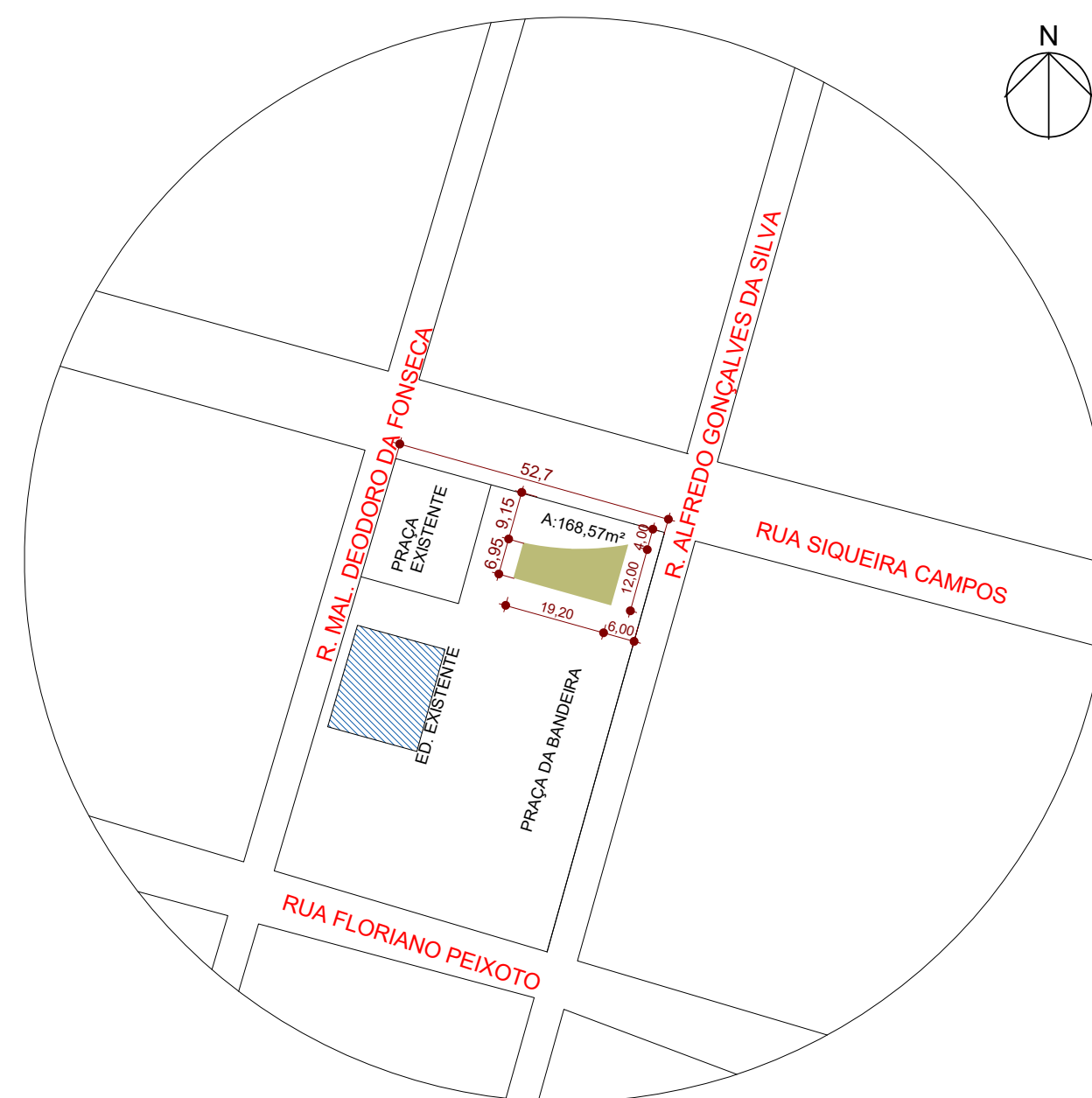
6 PLANTA DE LOCAÇÃO ESCALA -1 : 1250
