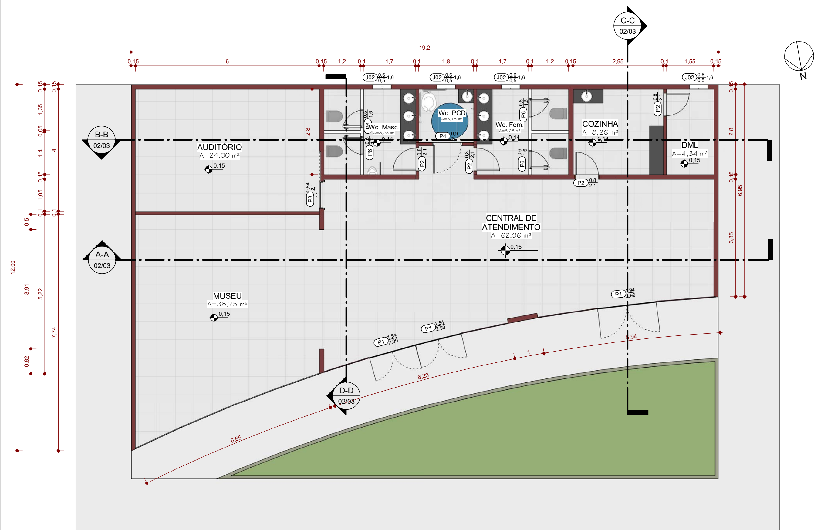
1 PLANTA BAIXA TÉRREO ESCALA -1 : 75
