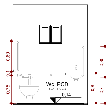
4 DETALHAMENTO PCD ESCALA - 1 : 50
