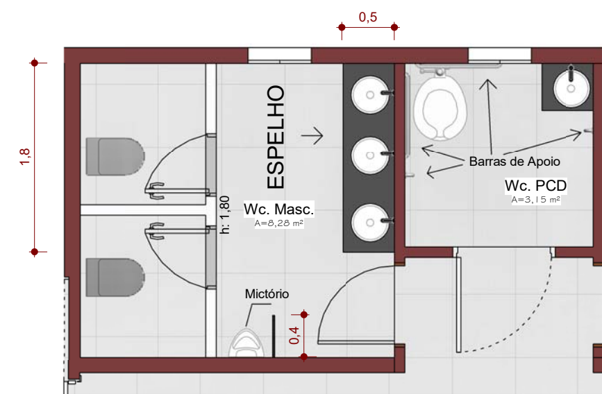
3 DETALHAMENTO BANHEIRO ESCALA - 1 : 50
