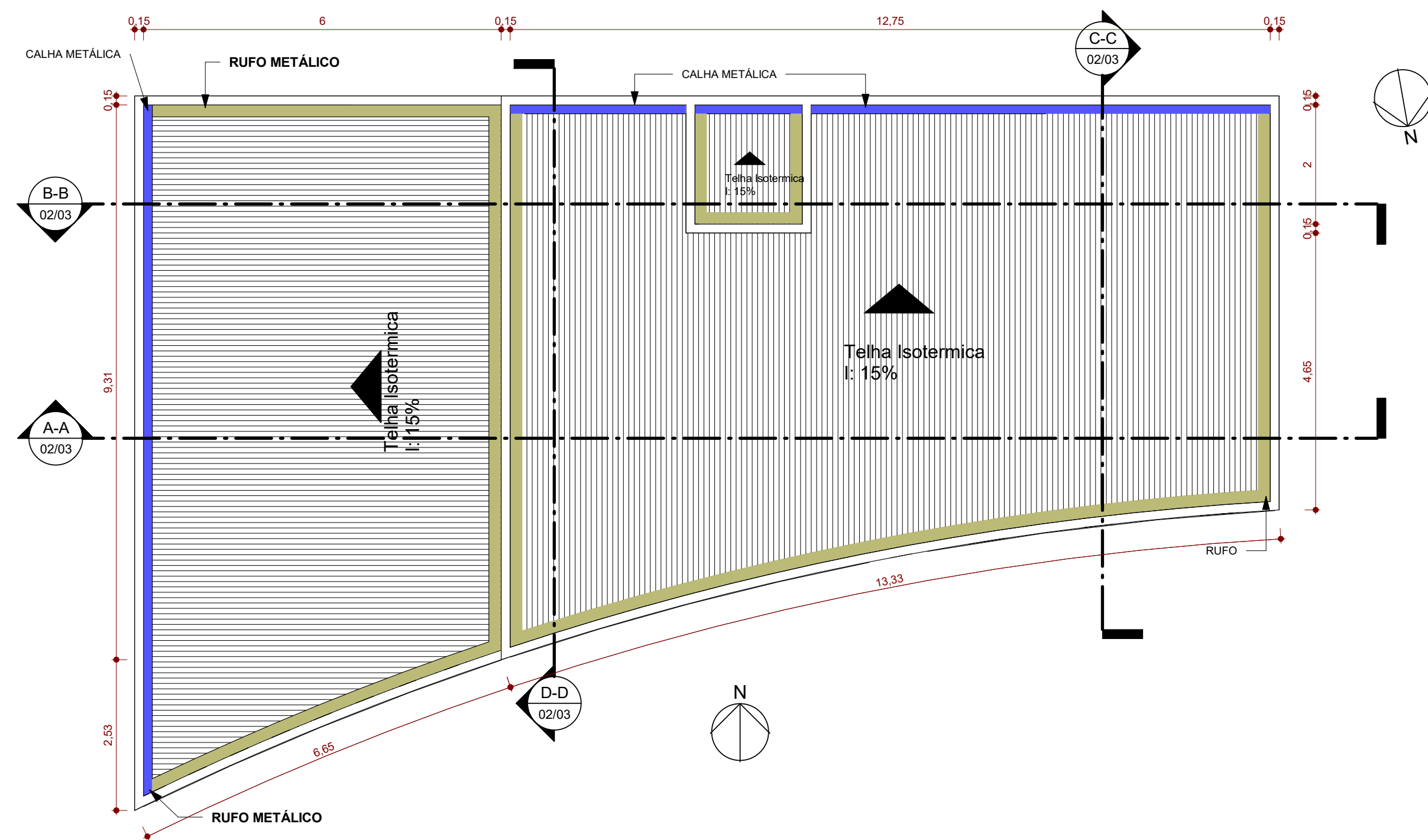
5 PLANTA BAIXA COBERTURA ESCALA -1 : 75
