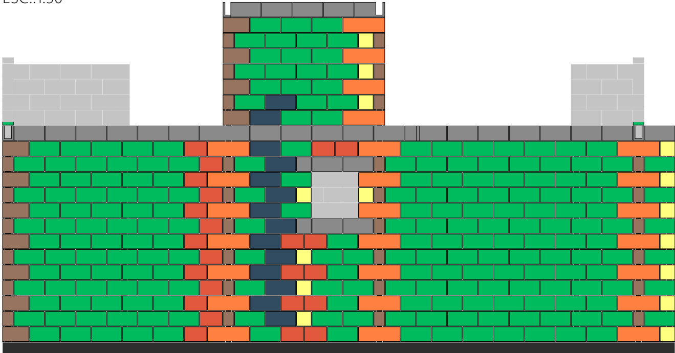
FACHADA 4 ESC.:1:50
