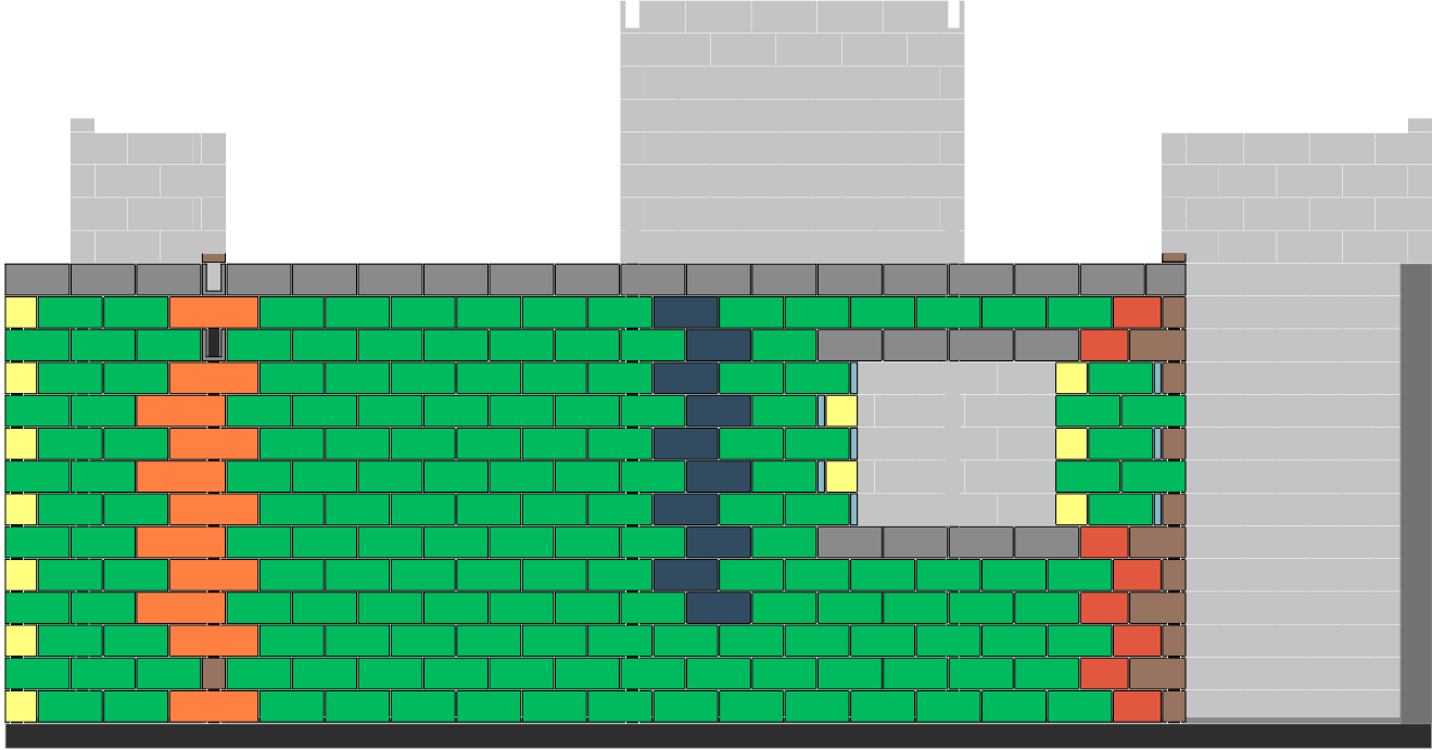
FACHADA 2 ESC.:1:50
