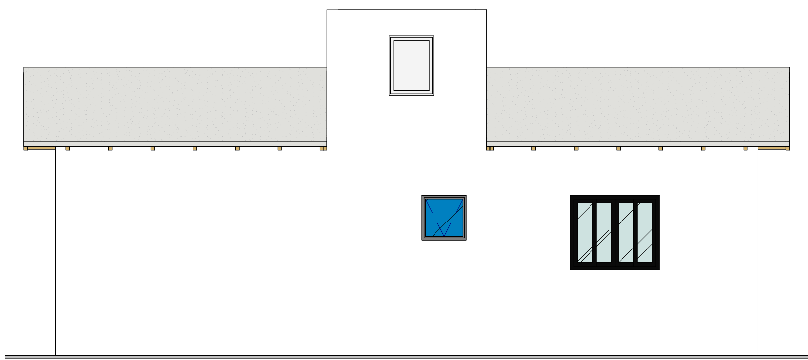
ELEVACÃO ESQUERDA 1 : 50
