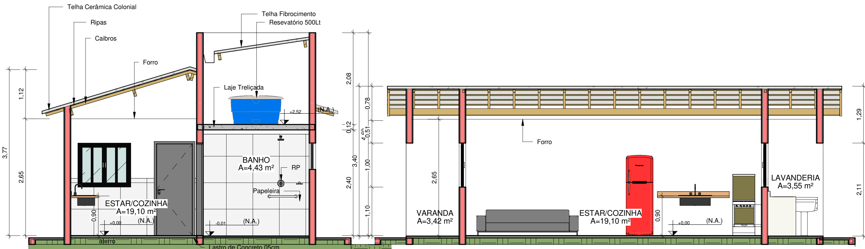
B-B 1 : 50
