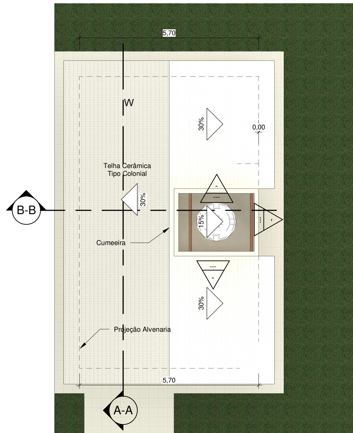
COBERTURA 1 : 75
