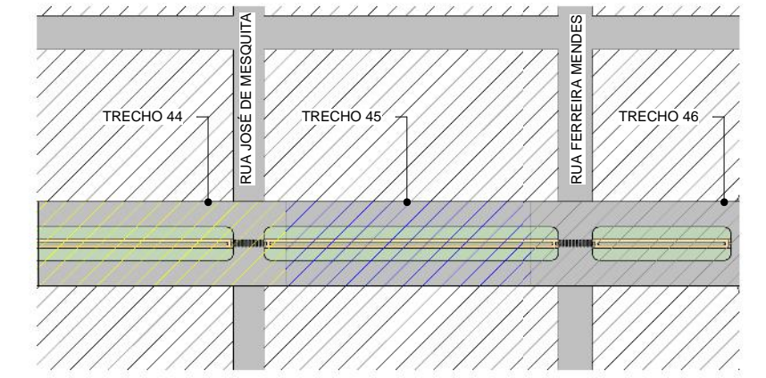
4 CROQUI ESQUEMÁTICO - 44,45,46 1 : 4000
