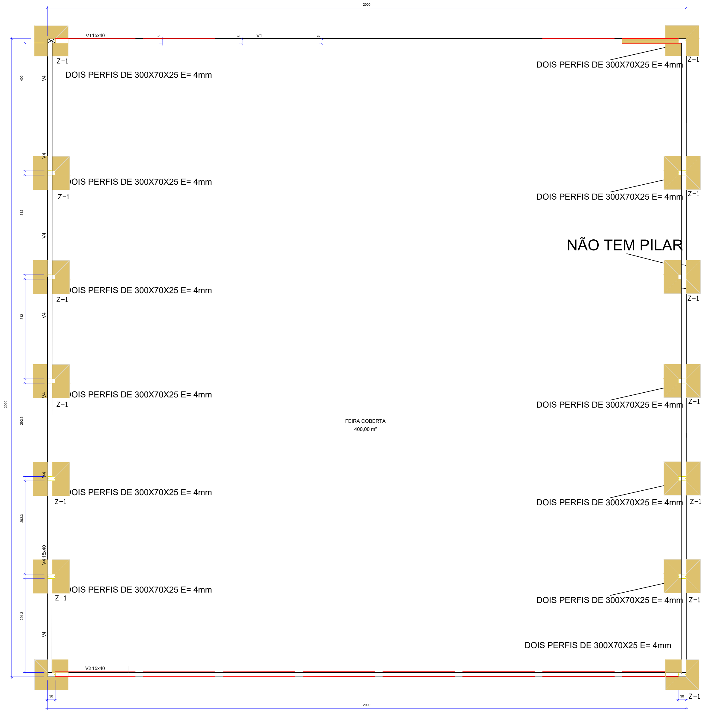
FORMA DO PAVIMENTO VIGA BALDRAME (NÍVEL 0) Escala 1:50
