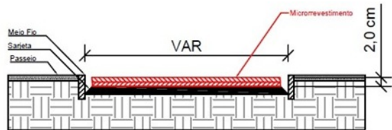
Figura 04 – Esquema de perfil transversal para Microrrevestimento.
