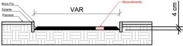
Figura 01 – Esquema de perfil transversal para reparo superficial.
