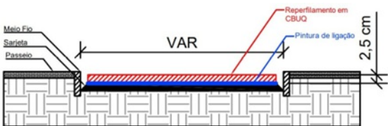
Figura 05 – Esquema de perfil transversal para reperfilamento em CBUQ.
