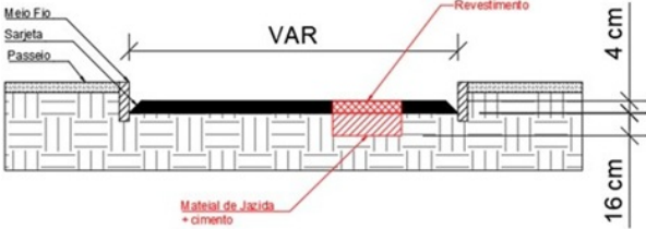
Figura 02 – Esquema de perfil transversal para reparo profundo.
