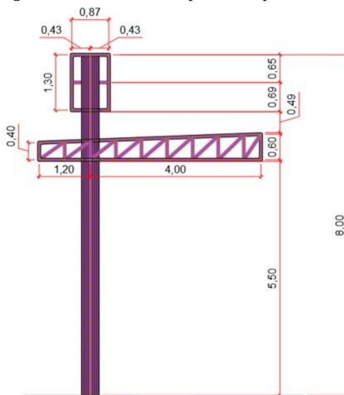
Figura 2 - Vista Frontal semipórtico simples
