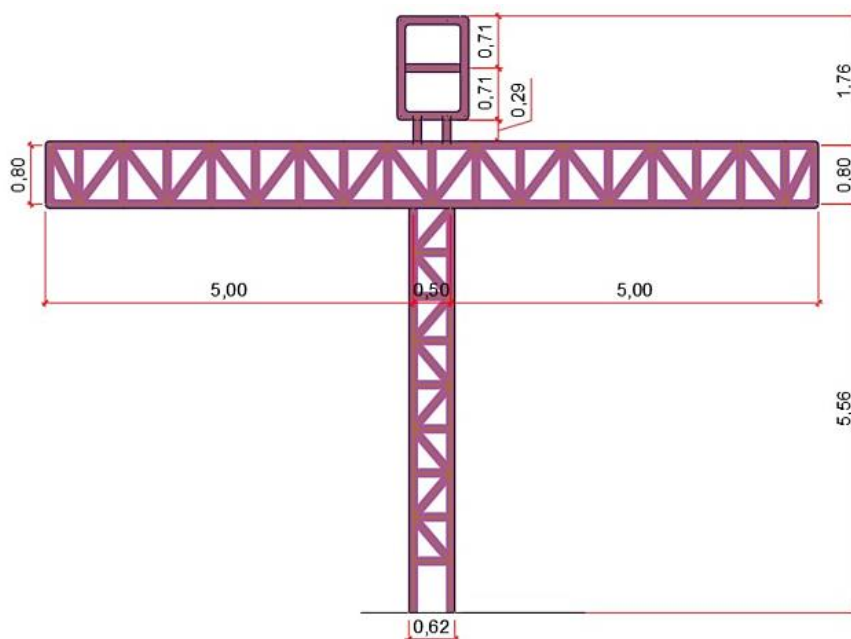
Figura 3 - Vista frontal semipórtico bilateral
