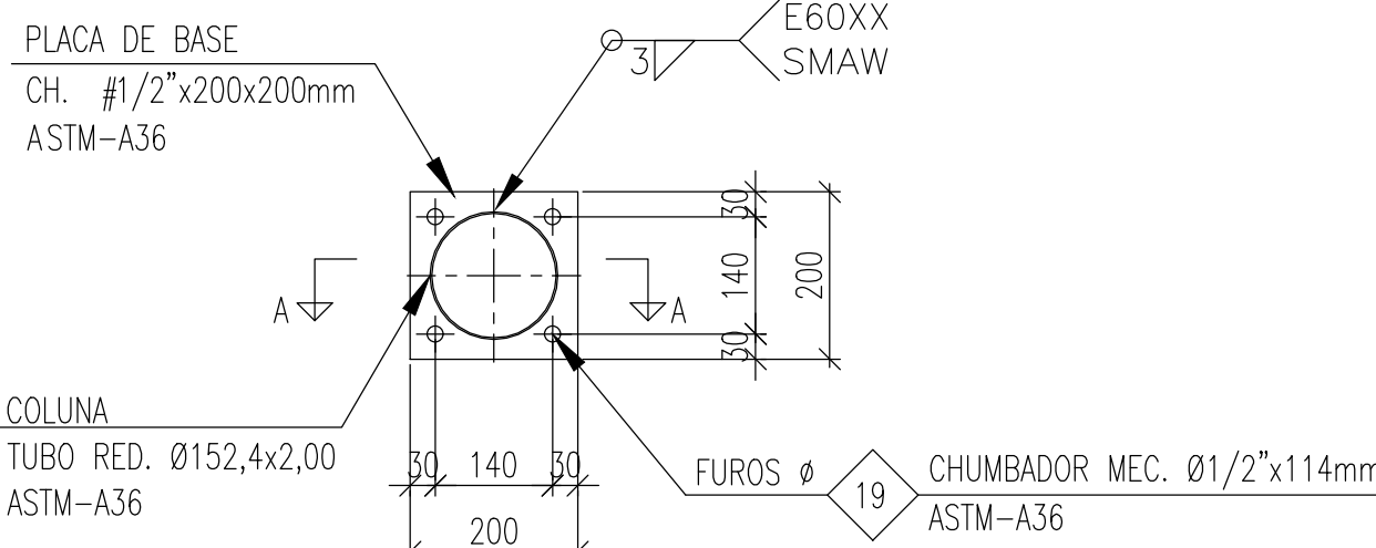
DET. 01 - PLACA DE BASE (CH. 01) ESCALA 1:10
