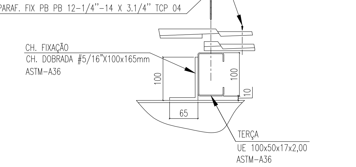
CORTE E-E (TERÇA UE 100x50x17x2,00) ESCALA 1:5
