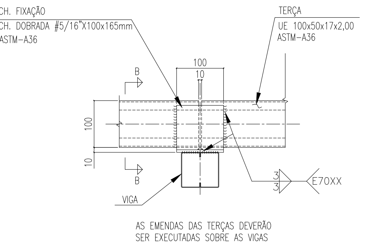
DET. 02 (TIP.) - FIXAÇÃO DAS TERÇAS ESCALA 1:5
