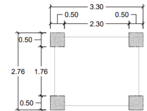
PLANTA BASE MODULAR (3000 X 2440)
