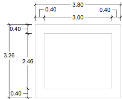
MODELO PASSEIO MODULAR (3000X2440)
