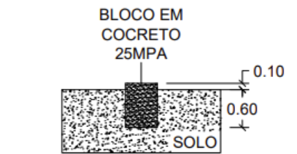
CORTE BLOCO MODULAR (3000X2440)
