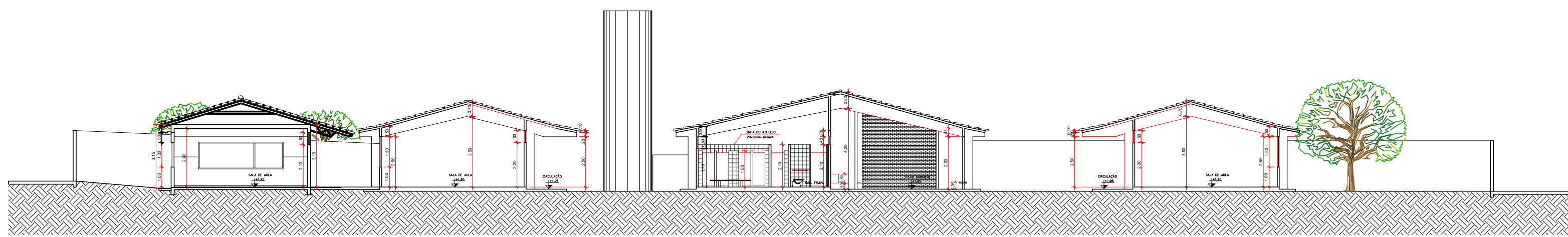
Corte AA Escala 1:175
