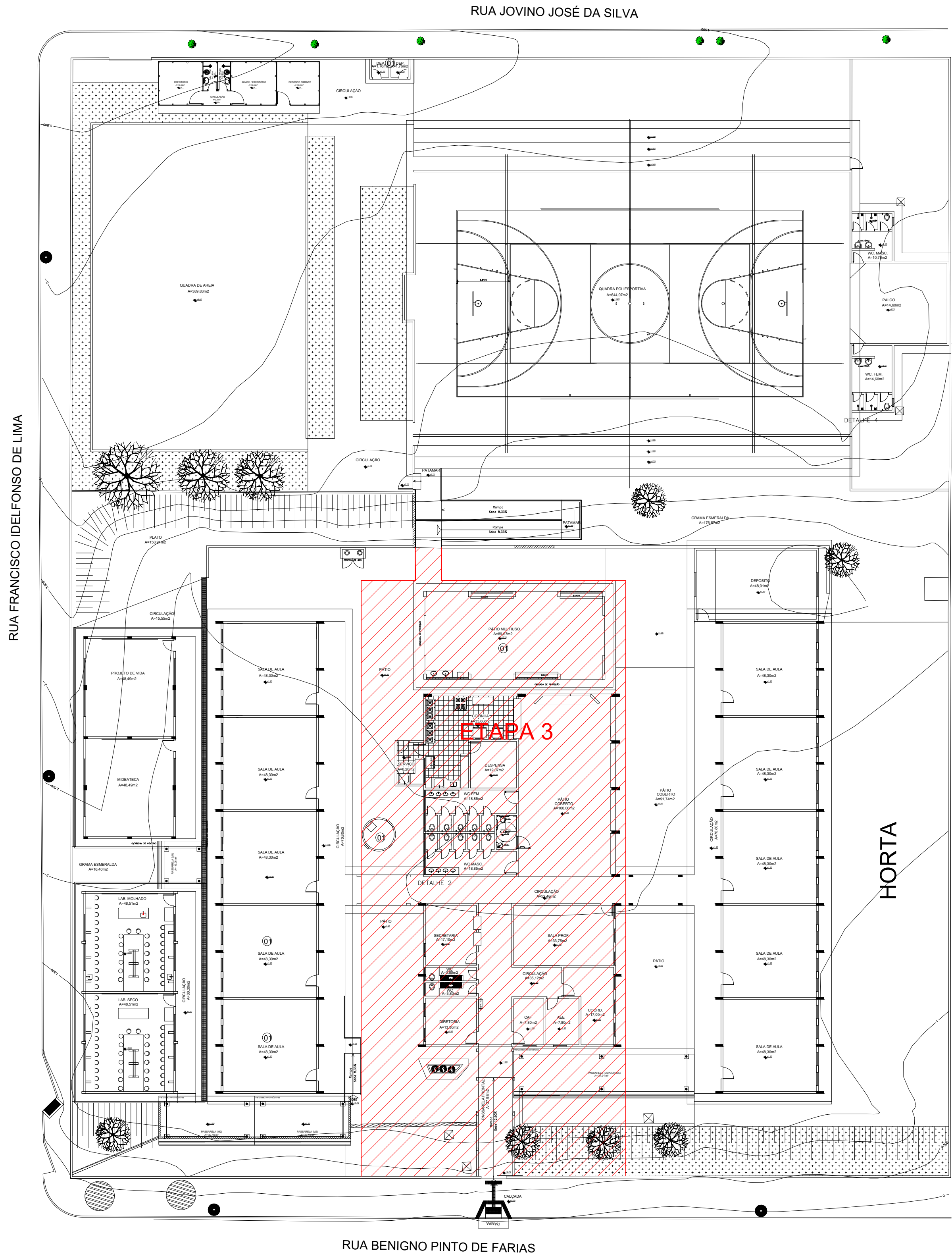
Panta Baixa - Tapume Escala 1:125
