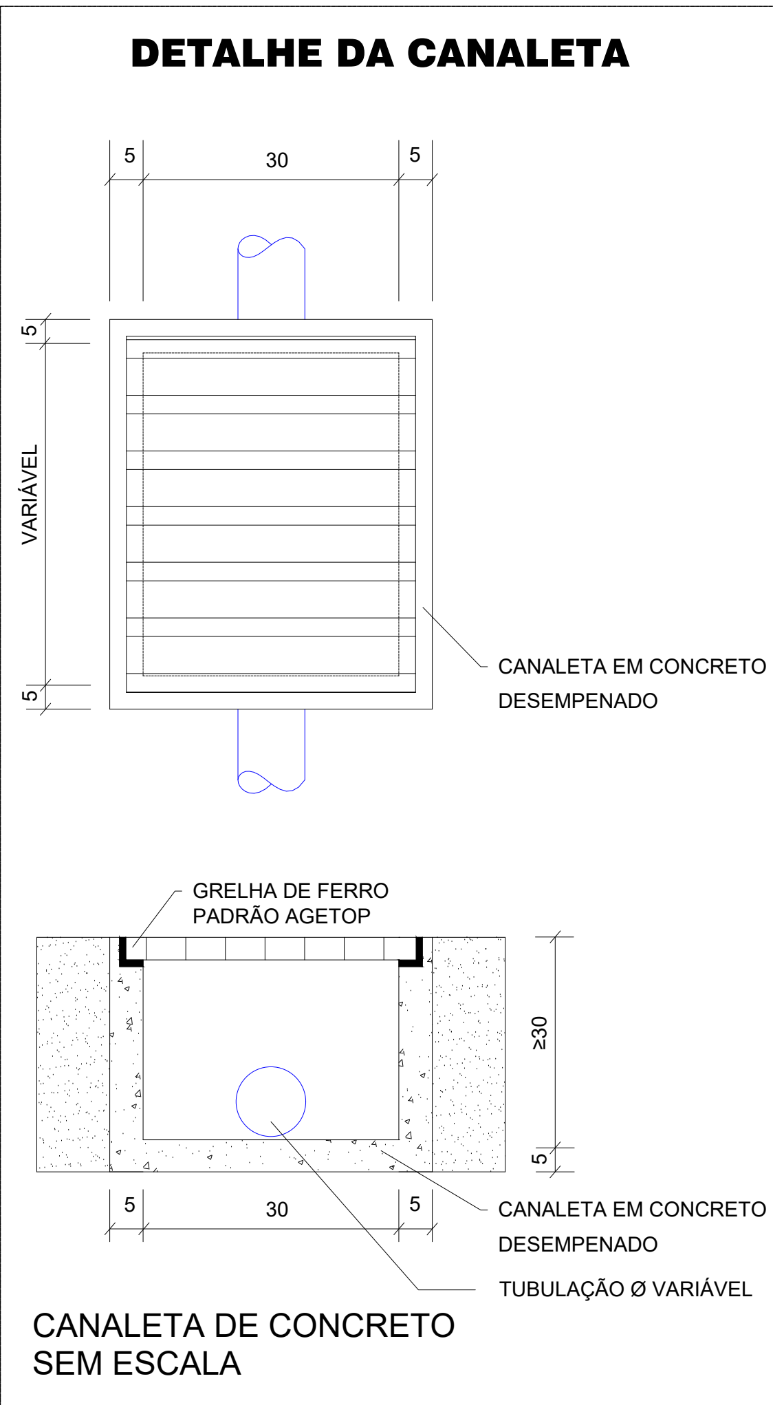
DETALHE H8 SEM ESCALA
