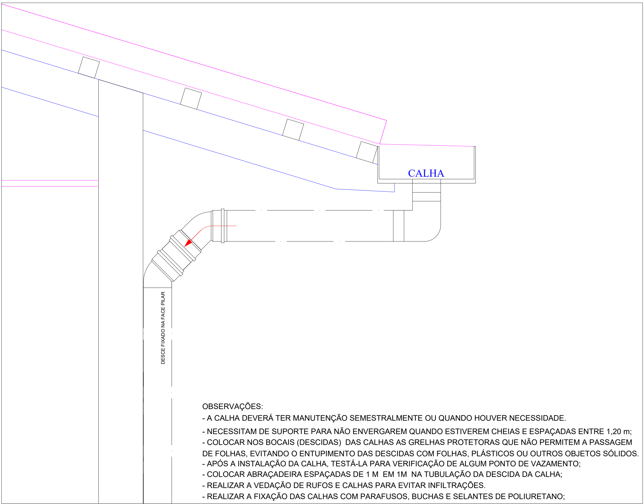
DETALHE DA CALHA SEM ESCALA
