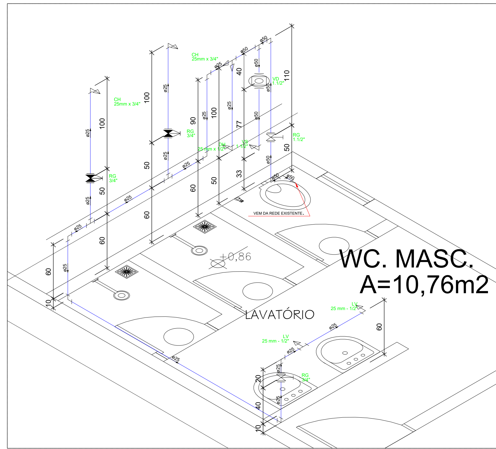
DETALHE H1 SEM ESCALA
