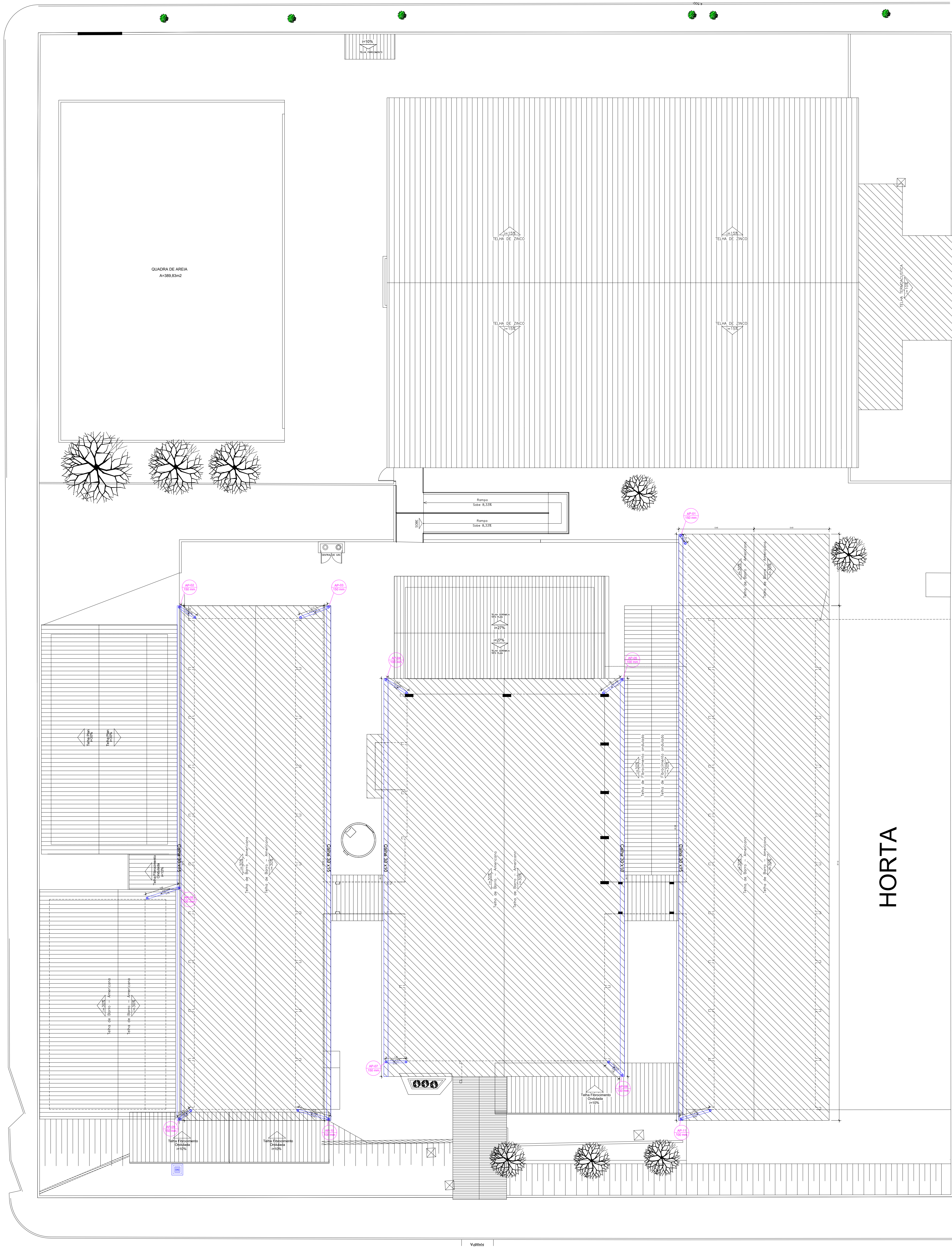
PLANTA BAIXA - ÁGUA PLUVIAL ESCALA 1:125
