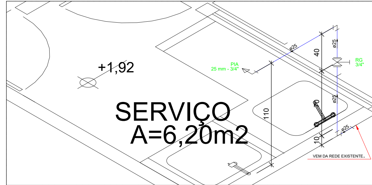
DETALHE H3 SEM ESCALA
