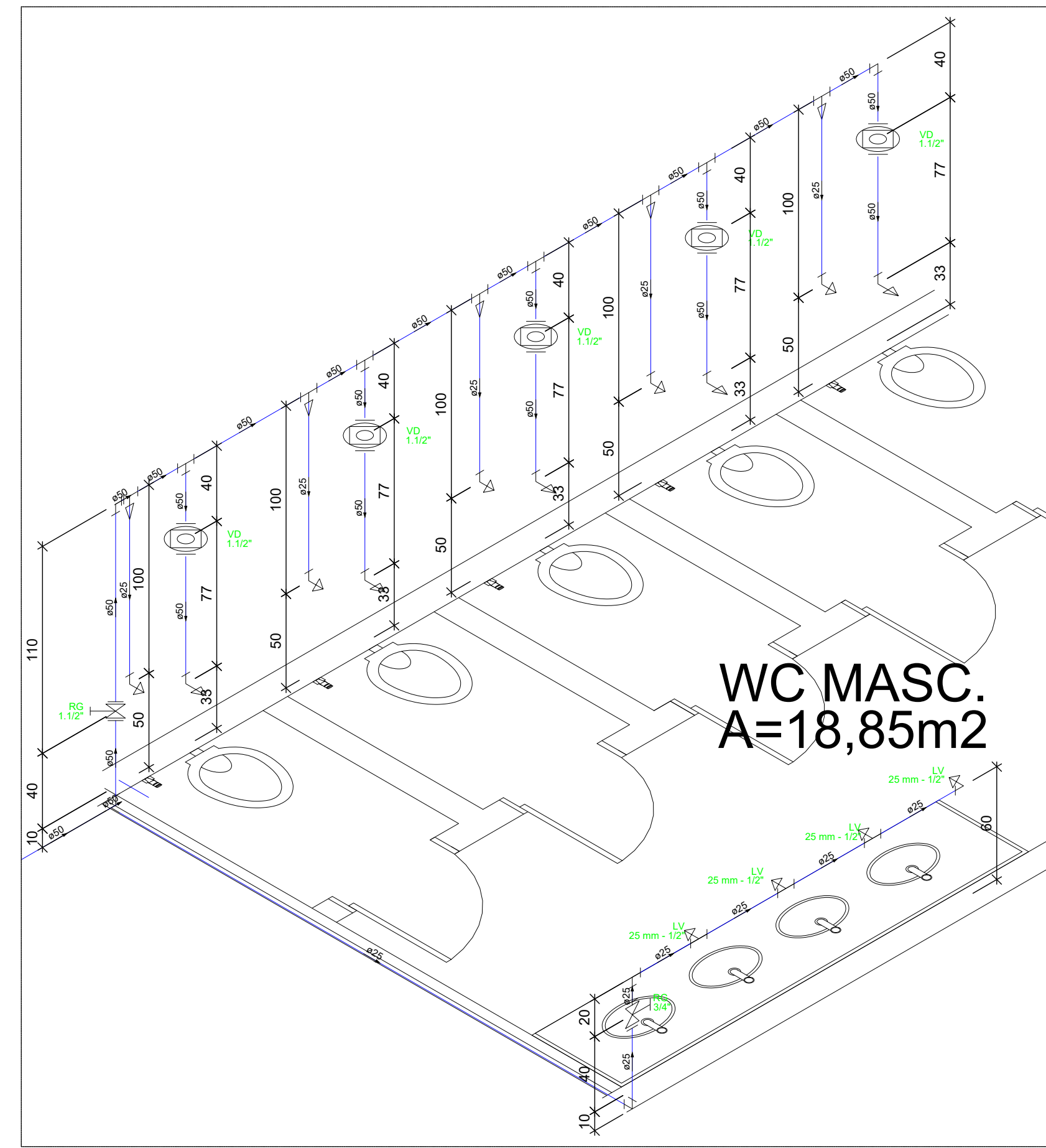
DETALHE H7 SEM ESCALA
