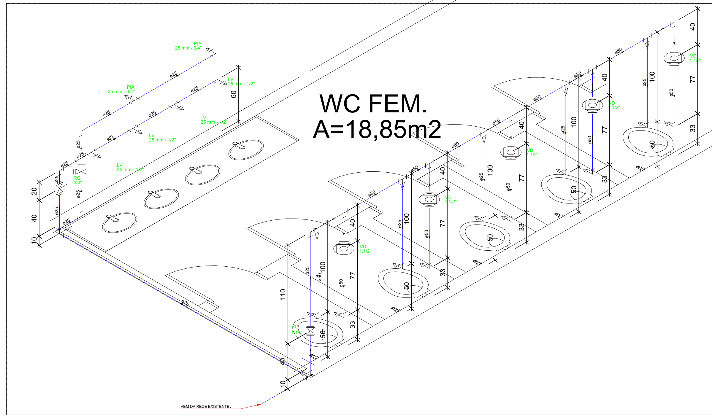
DETALHE H5 SEM ESCALA
