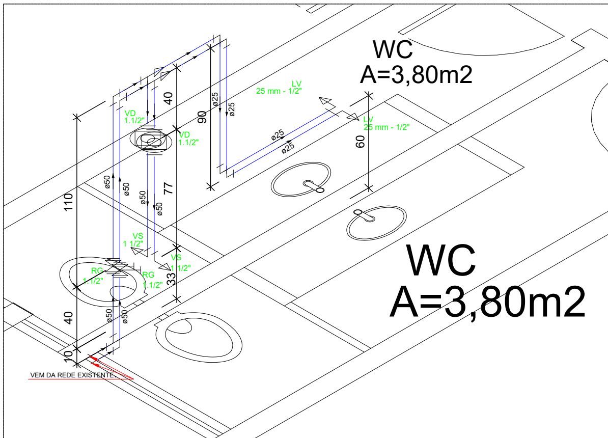
DETALHE H9 SEM ESCALA
