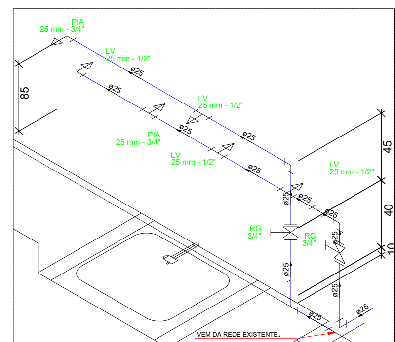
DETALHE H4 SEM ESCALA
