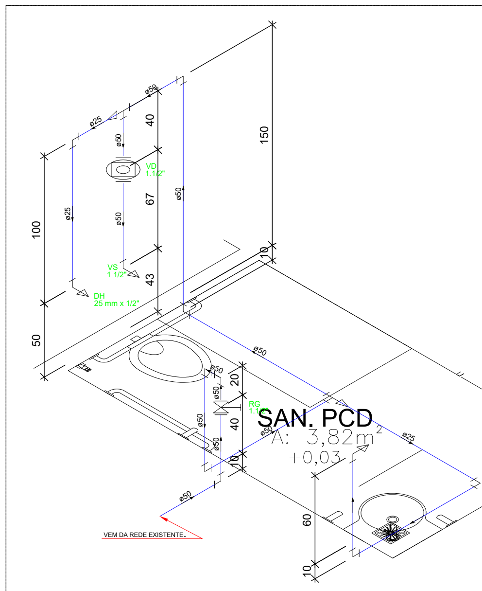
DETALHE H6 SEM ESCALA
