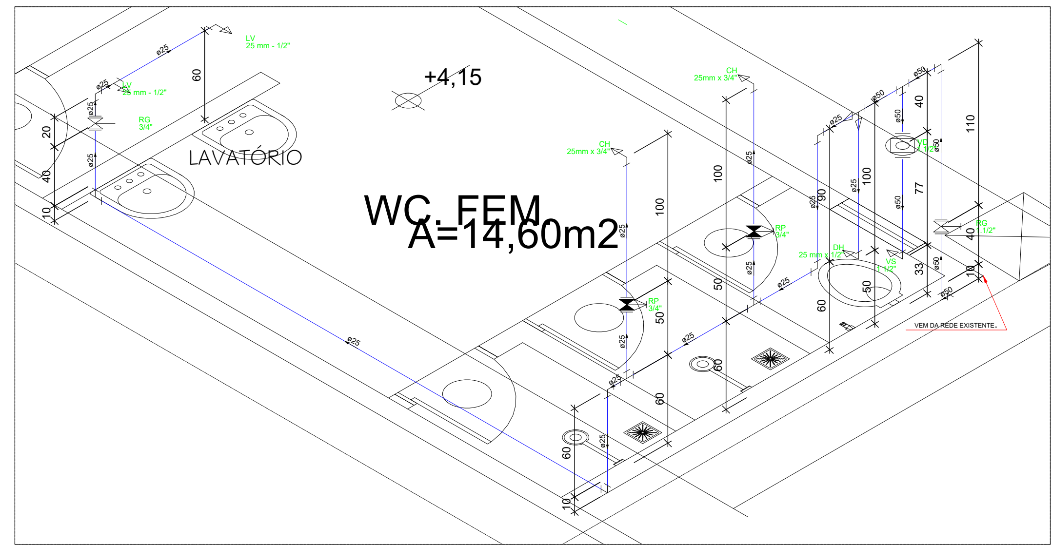
DETALHE H2 SEM ESCALA
