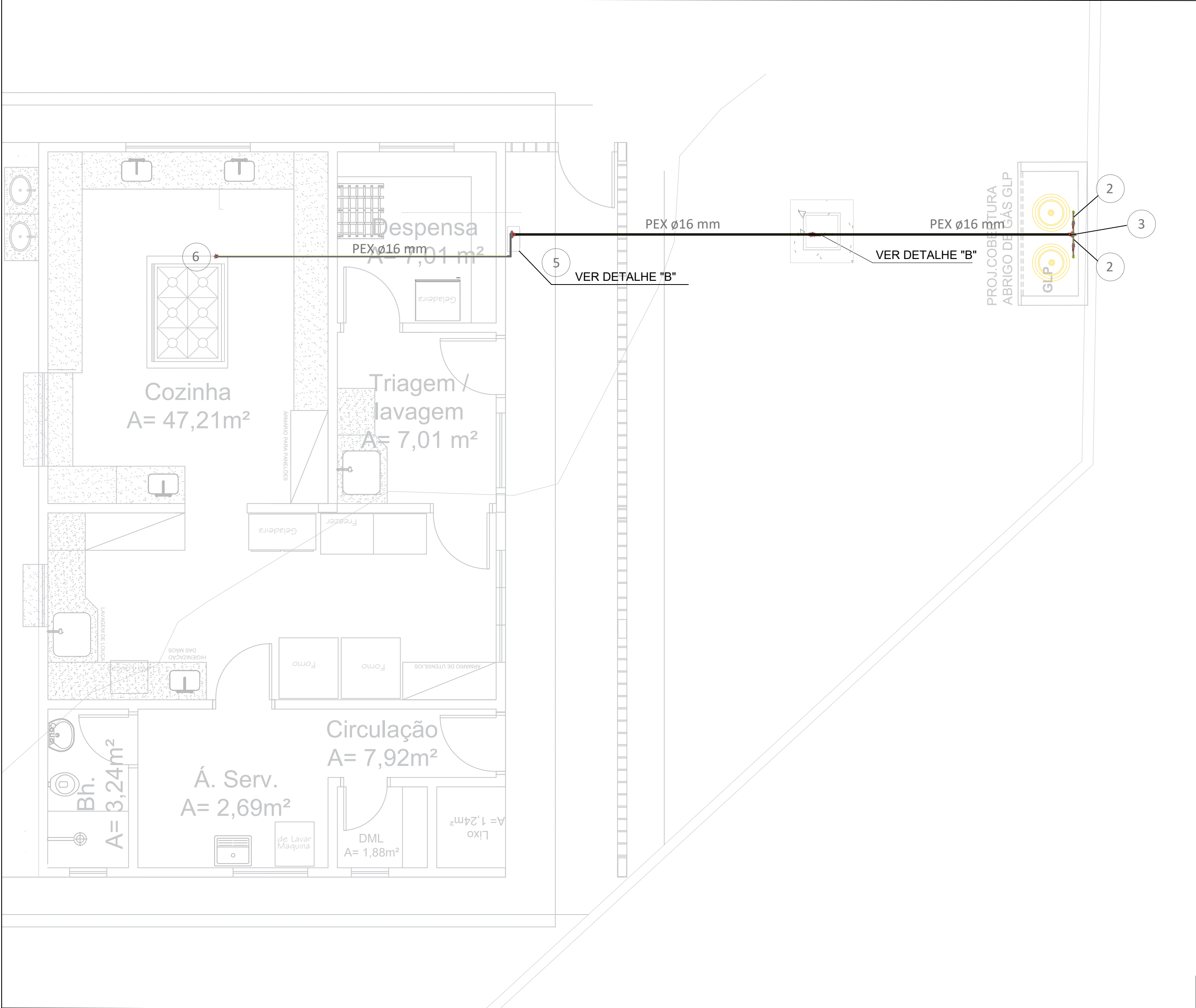
PLANTA BAIXA SETORIZAÇÃO COZINHA Escala 1:50
