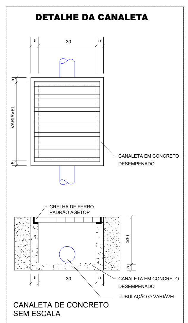
DETALHE DA CANALETA
