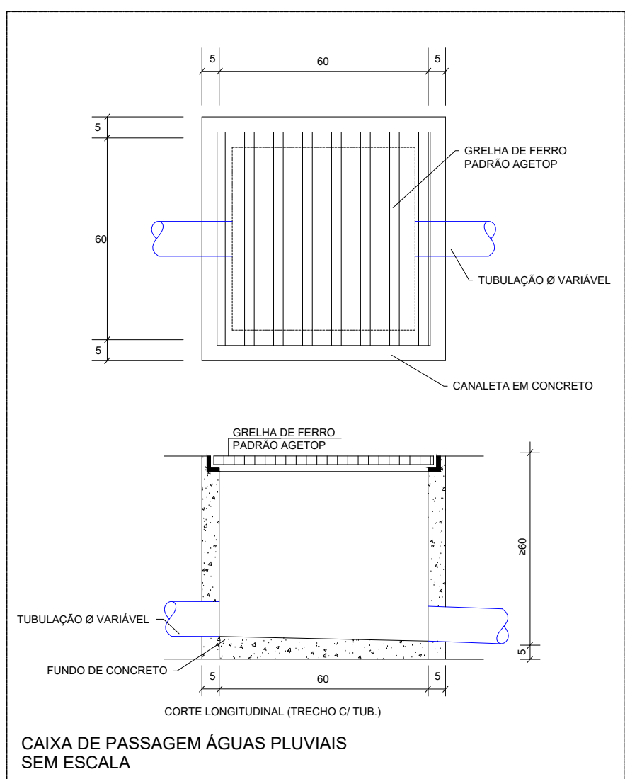
CAIXA DE PASSAGEM ÁGUAS PLUVIAIS SEM ESCALA
