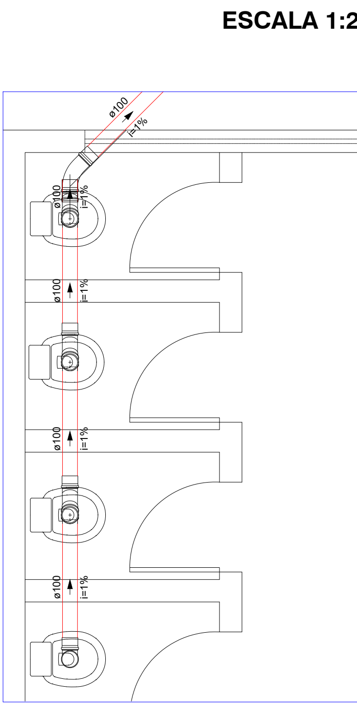
PLANTA BAIXA - ESGOTO E DRENAGEM ESCALA 1:100
