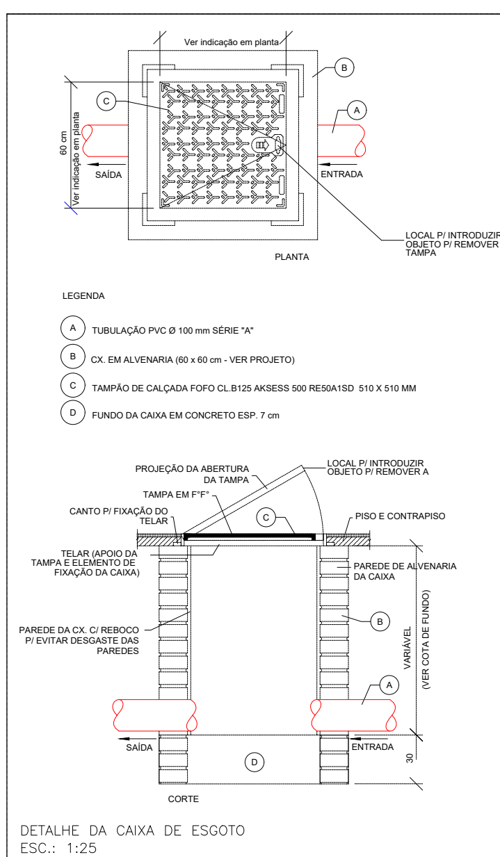
DETALHE DA CAIXA DE ESGOTO ESCALA 1:25
