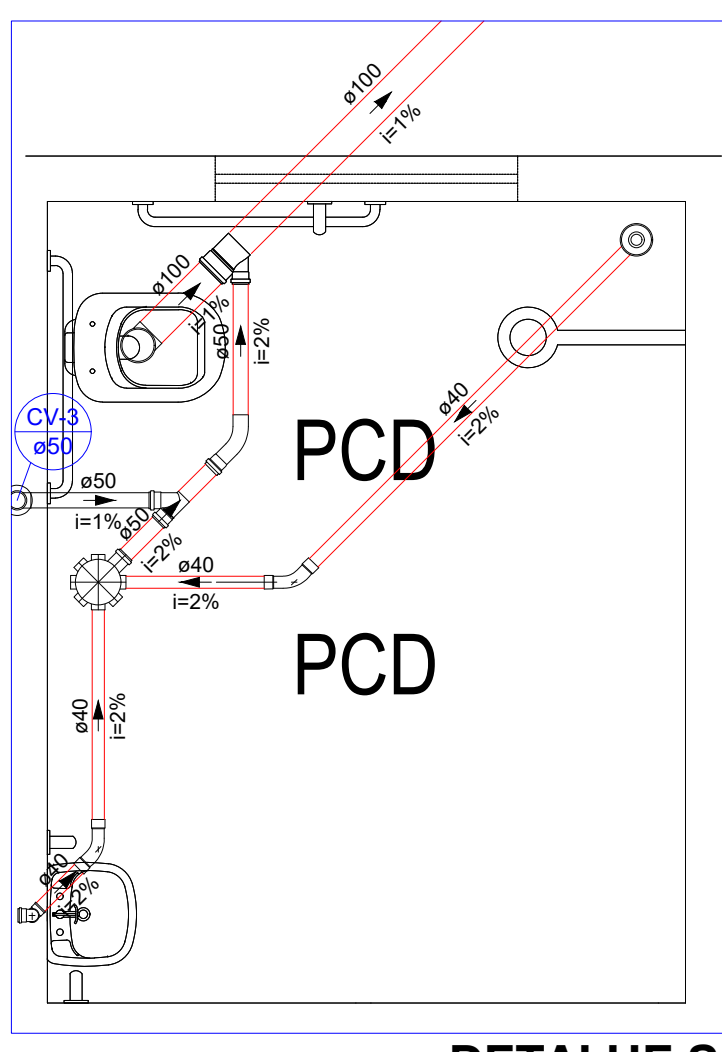
DETALHE S3 ESCALA 1:25
