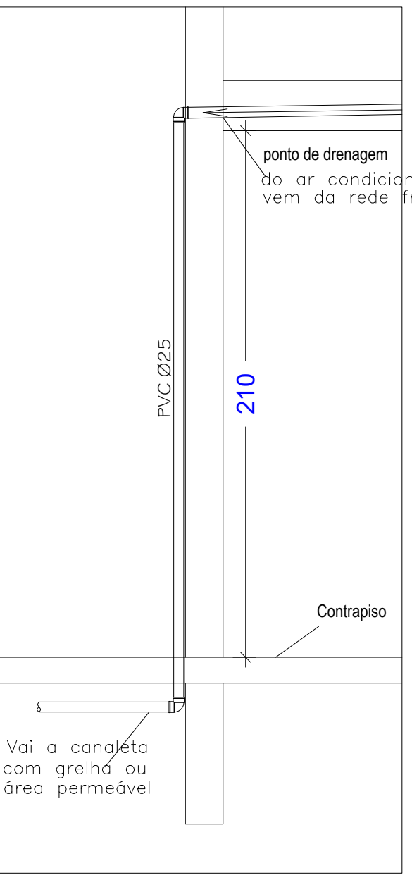
Corte Esquemático Dreno do Ar Condicionado Sem Escala
