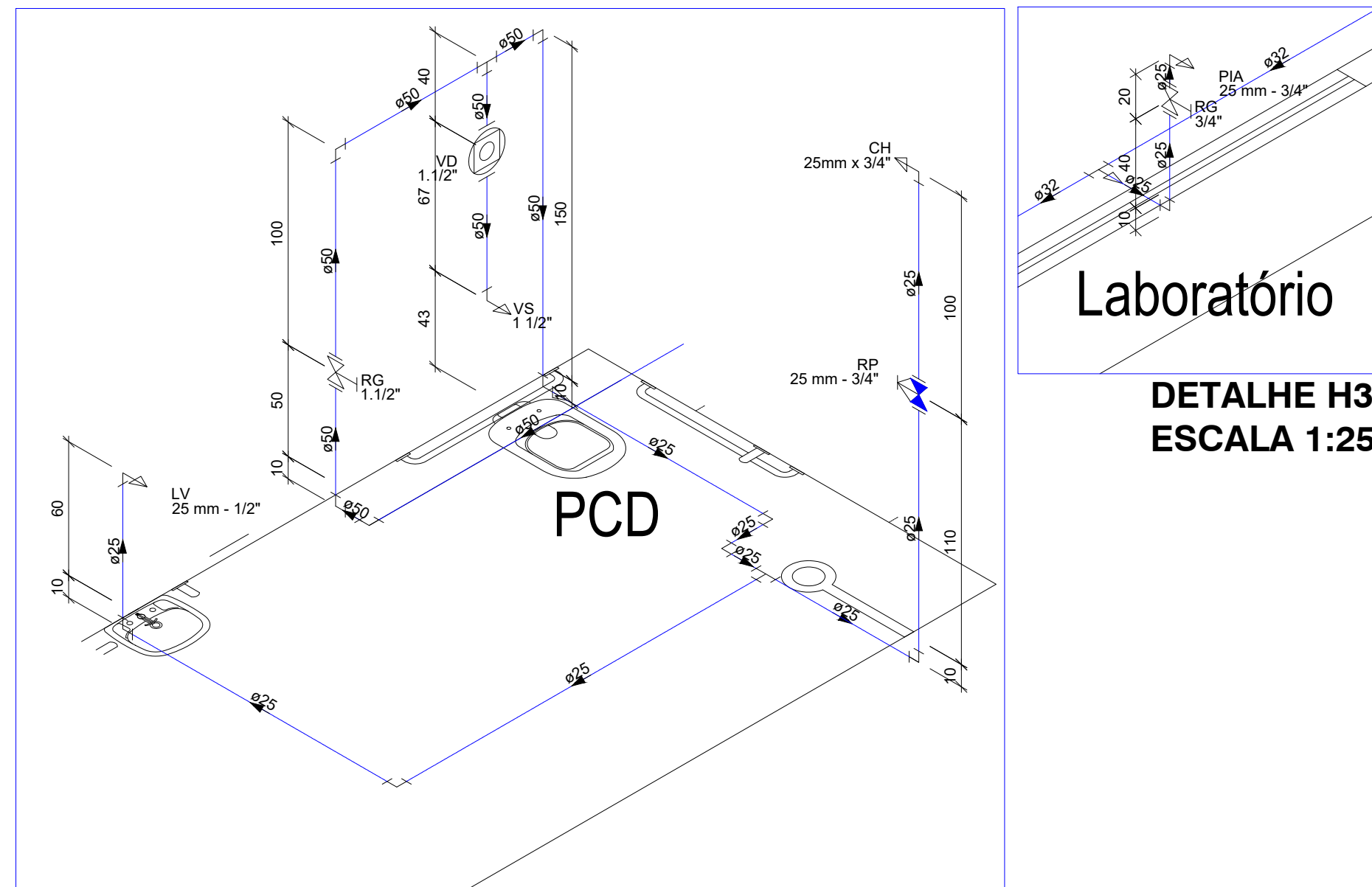
DETALHE H6 ESCALA 1:25
