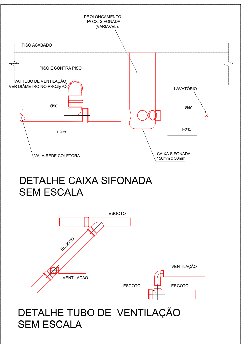
DETALHE CAIXA SIFONADA SEM ESCALA
