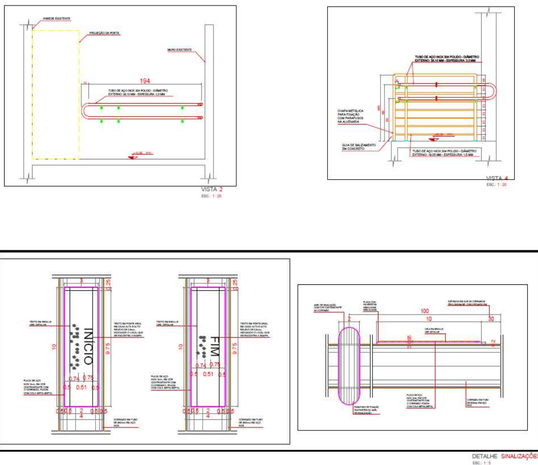
Figura 7: AURILÂNDIA – Projeto dos Corrimãos e Guarda-corpos
