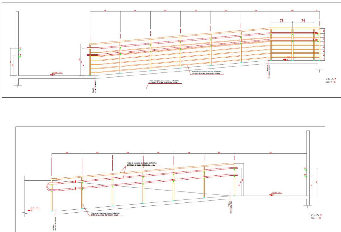
Figura 5: AURILÂNDIA – Projeto dos Corrimãos e Guarda-corpos
