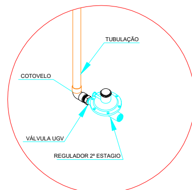
DETALHE "D" REGULADOR DE 2º ESTAGIO INSTALADO NAS PAREDES PROXIMA AOS PONTOS DE CONSUMO
