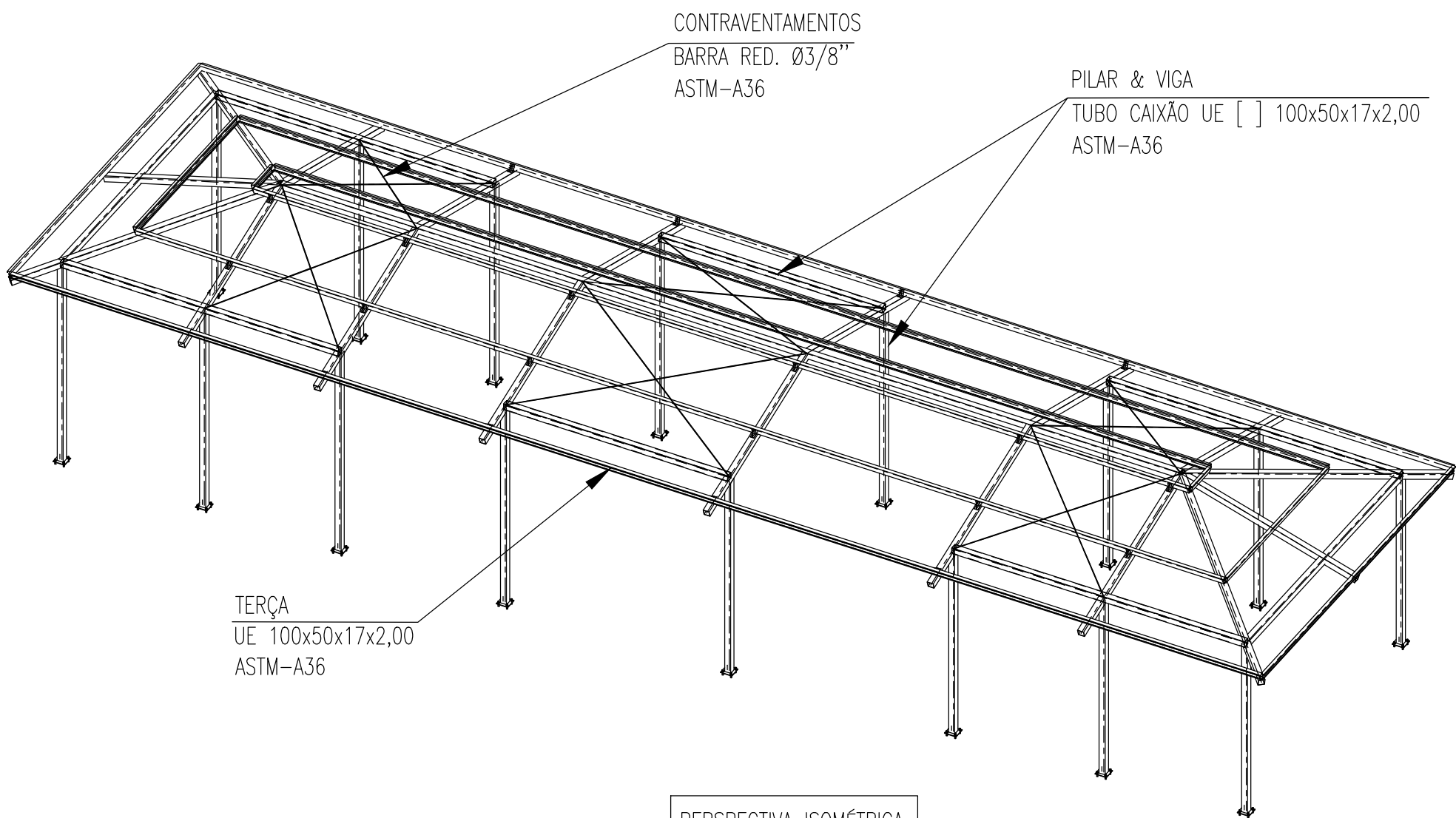
PERSPECTIVA ISOMÉTRICA SEM ESCALA
