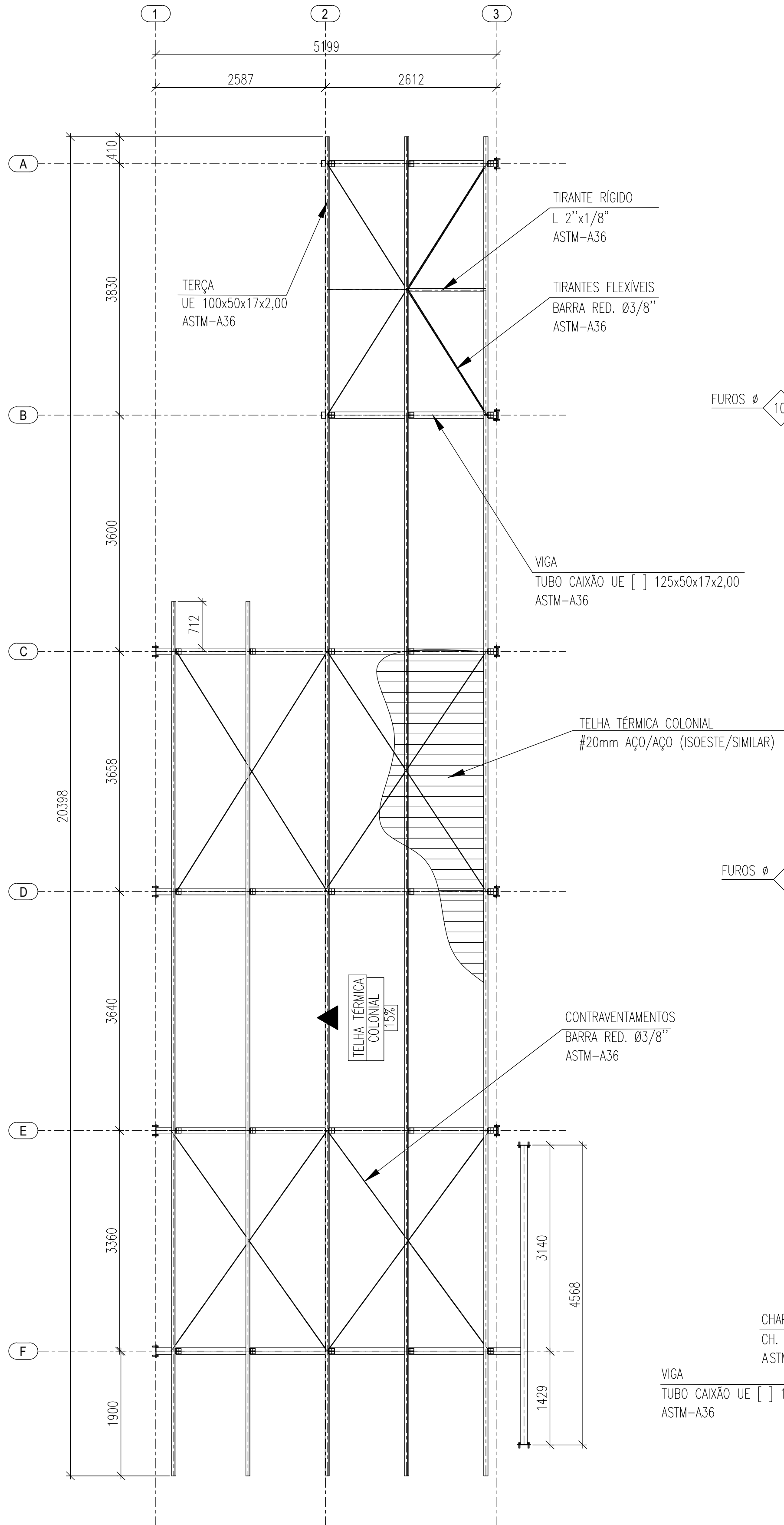
PLANO DE COBERTURA ESCALA 1:50
