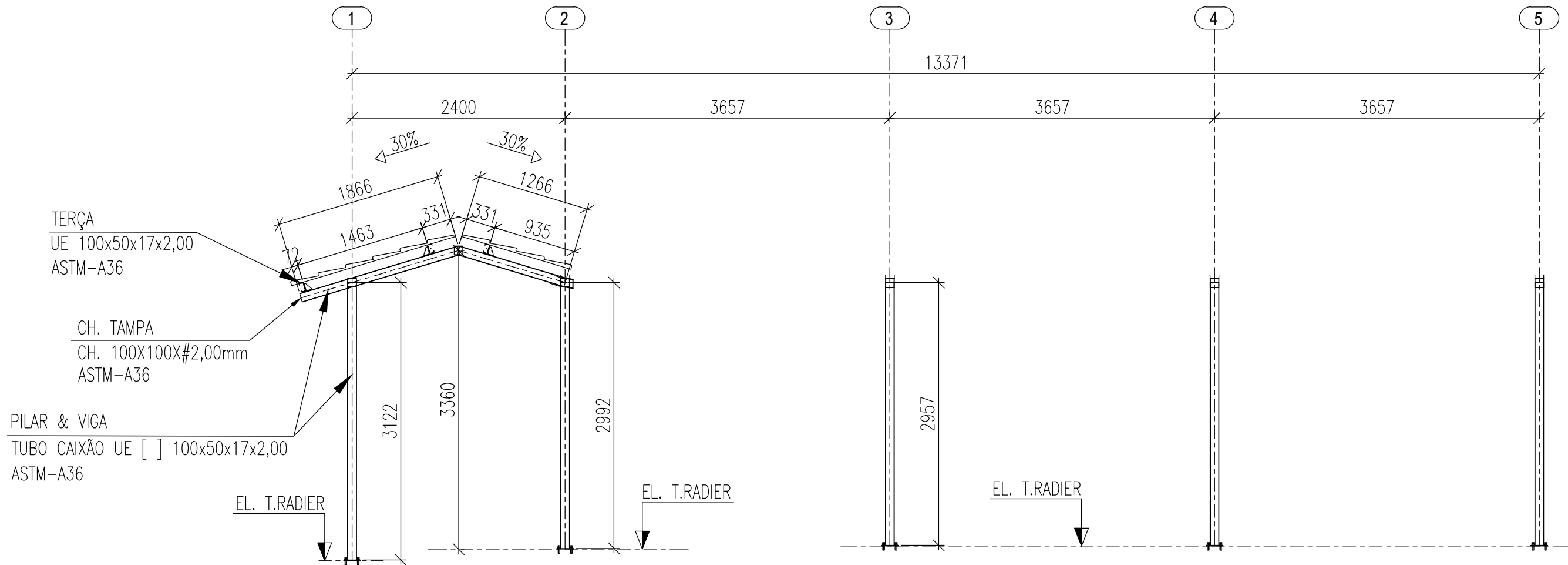
ELEVÇÃO FILA H ESCALA 1:50
