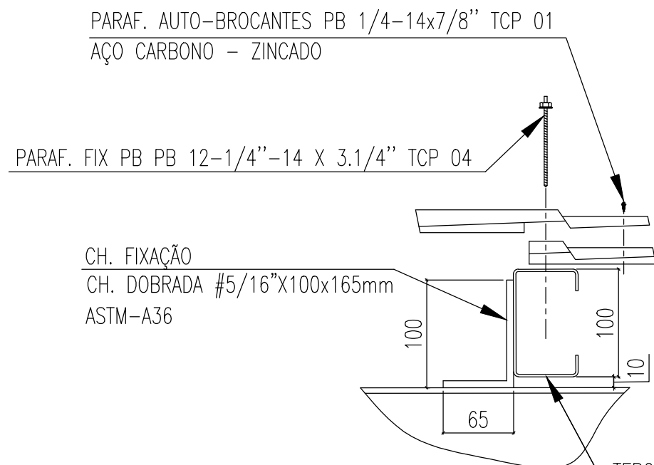
CORTE E-E (TERÇA UE 100x50x17x2,00) ESCALA 1:5
