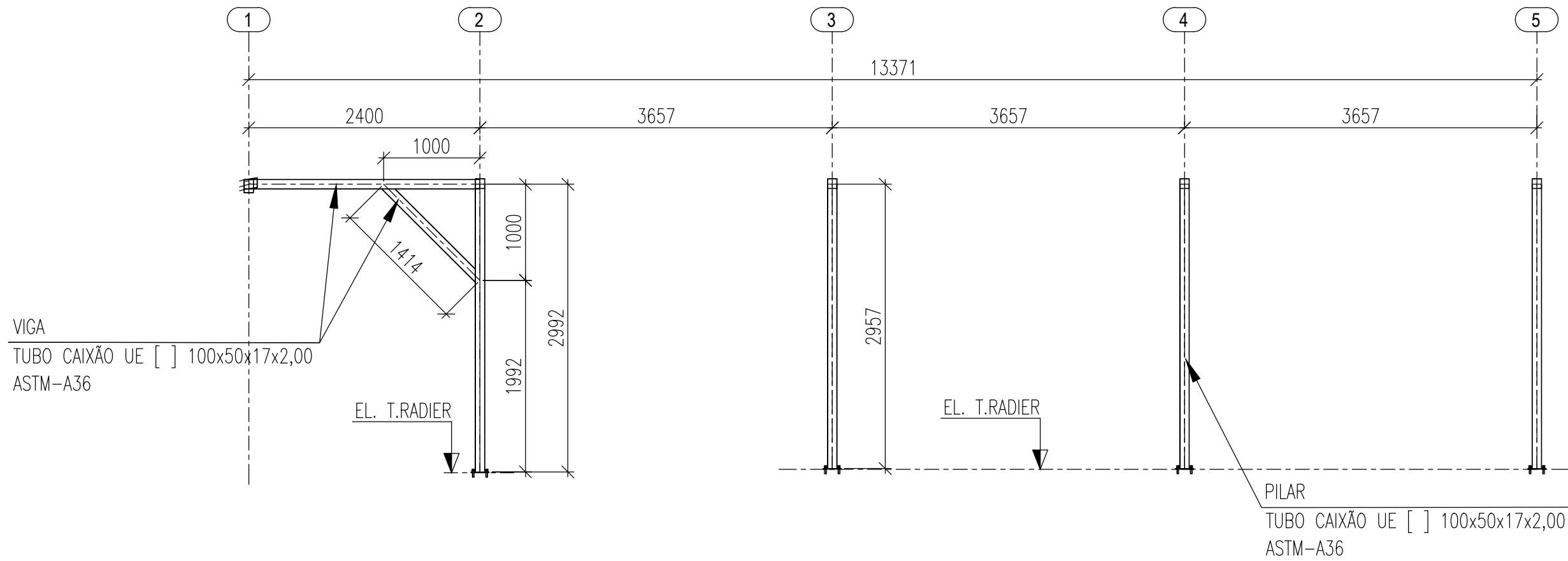
ELEVÇÃO FILA I ESCALA 1:50
