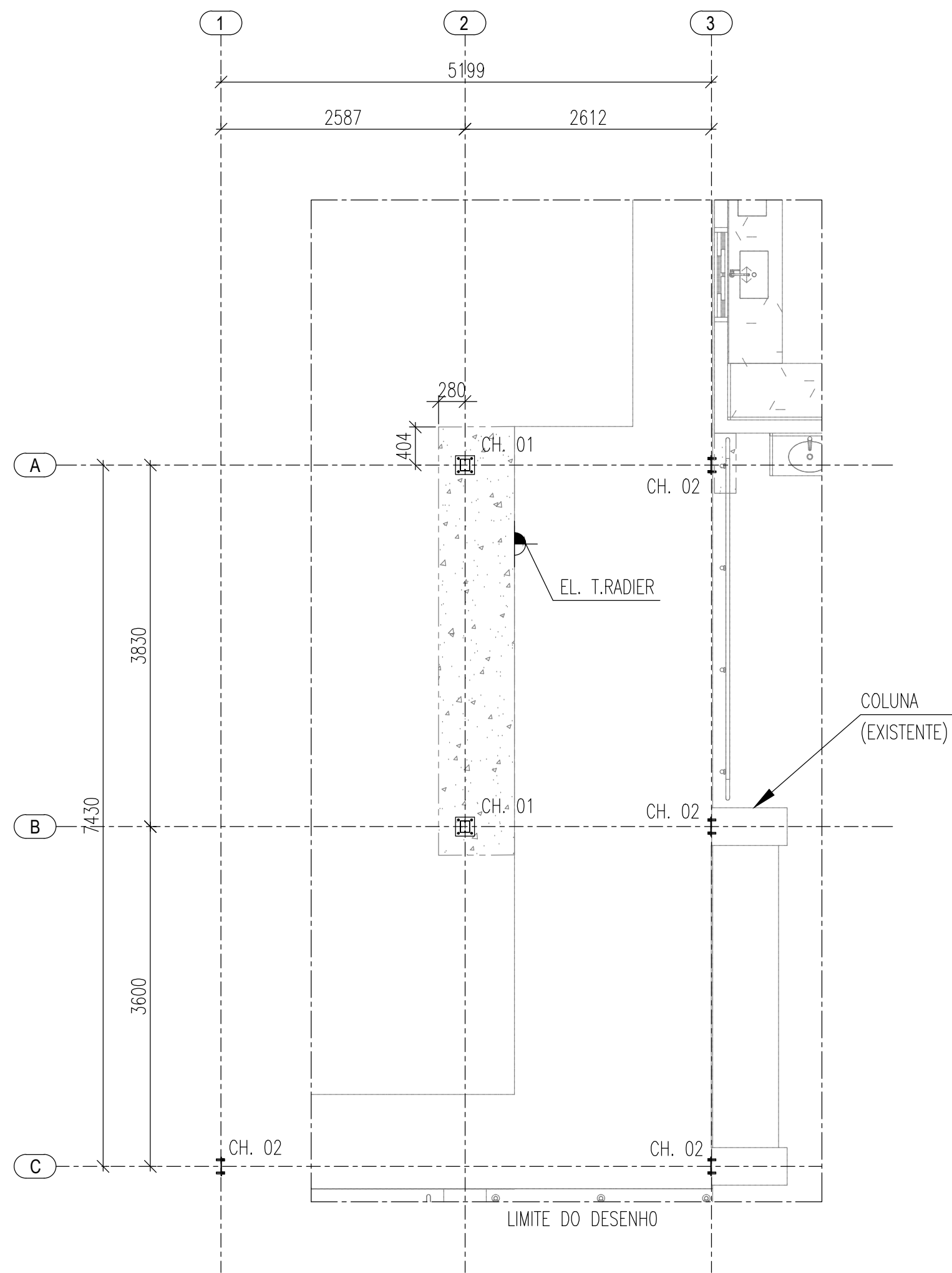
PLANO DE BASES ESCALA 1:50
