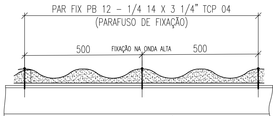
DETALHE TIP. - FIXAÇÃO DAS TELHAS SEM ESCALA
