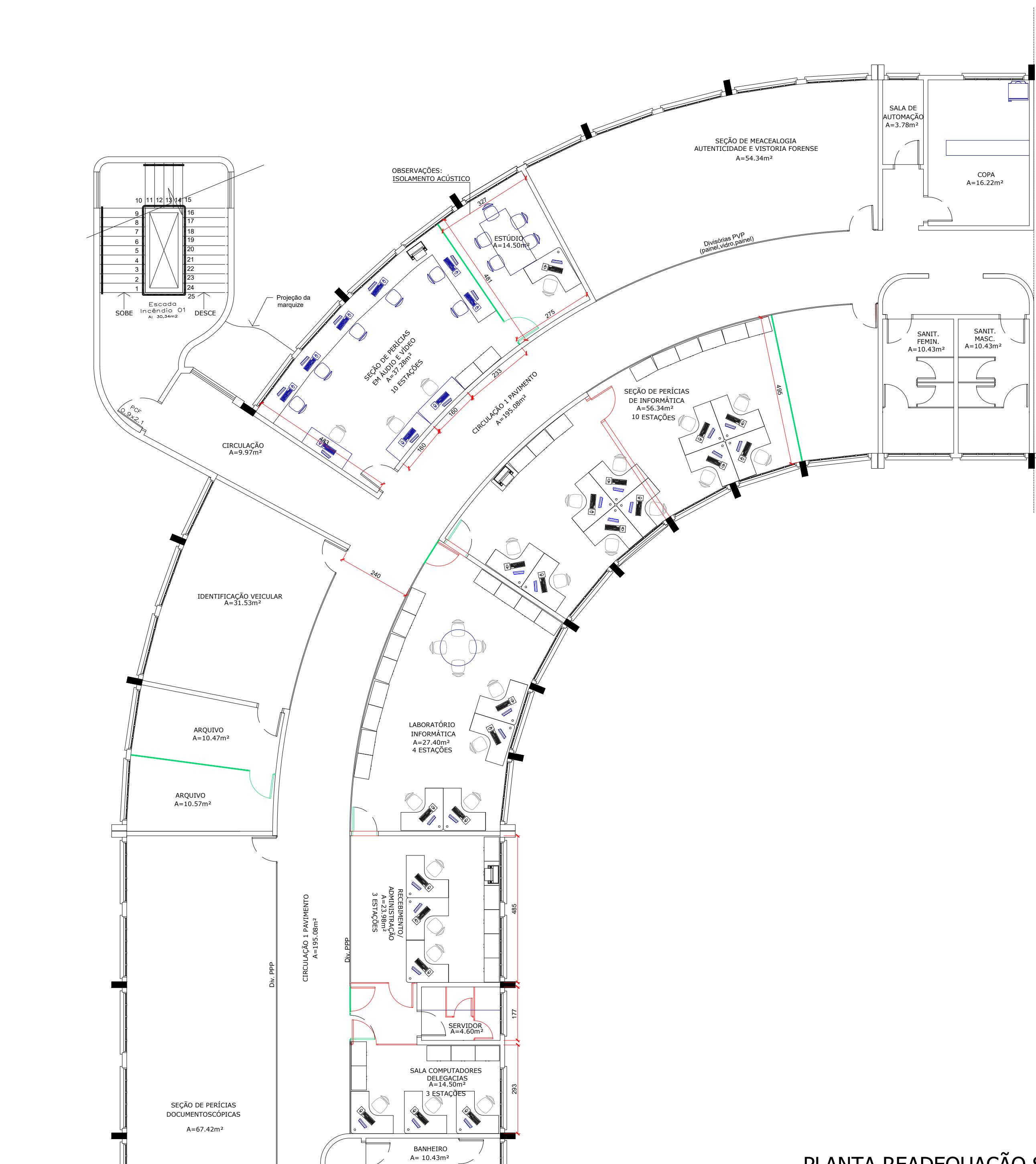
PLANTA READEQUAÇÃO SEÇÃO INFORMÁTICA/ PERÍCIAS EM ÁUDIO E VÍDEO escala: 1 : 100
