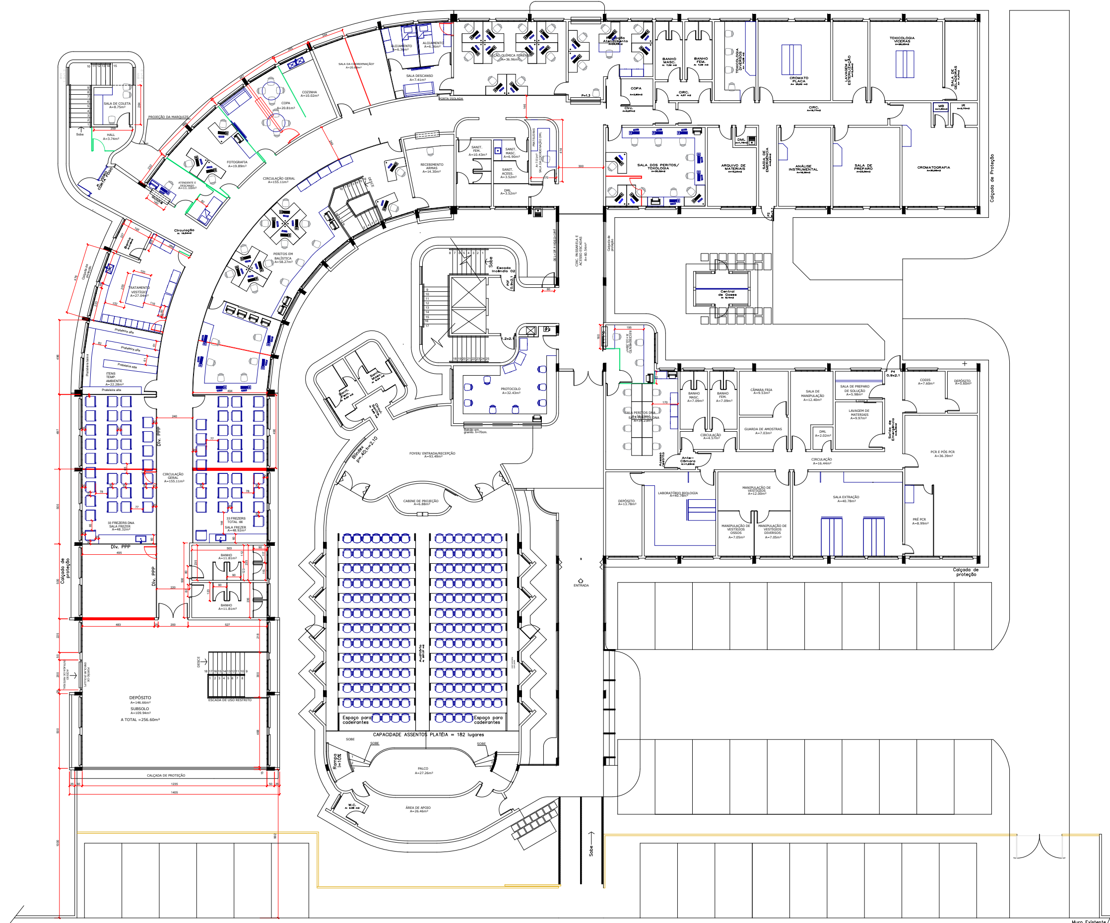
PLANTA PAVIMENTO TÉRREO sem escala
