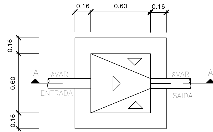
PLANTA BAIXA – CAIXA DE INSPEÇÃO (CI) ESCALA 1:25
