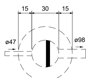
Caixa de gordura - TÉRREO Planta baixa - ESC. 1:25
