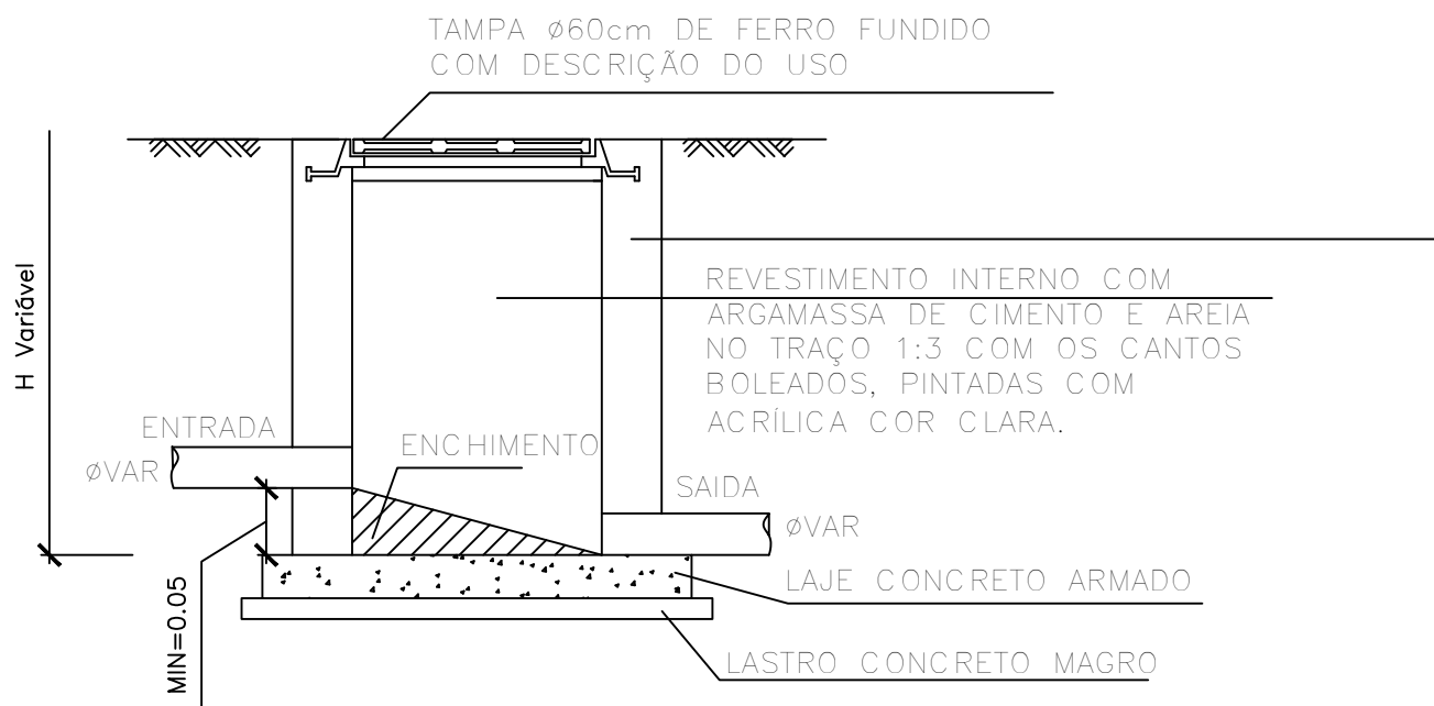
CORTE AA – CAIXA DE INSPEÇÃO (CI) ESCALA 1:25
