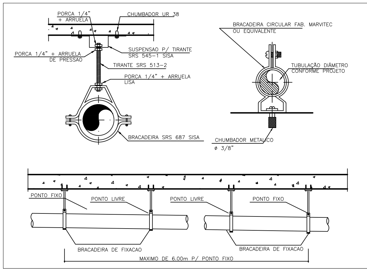
DETALHE 22 FISCAL DE DUTO APARENTE 90º ENCA
