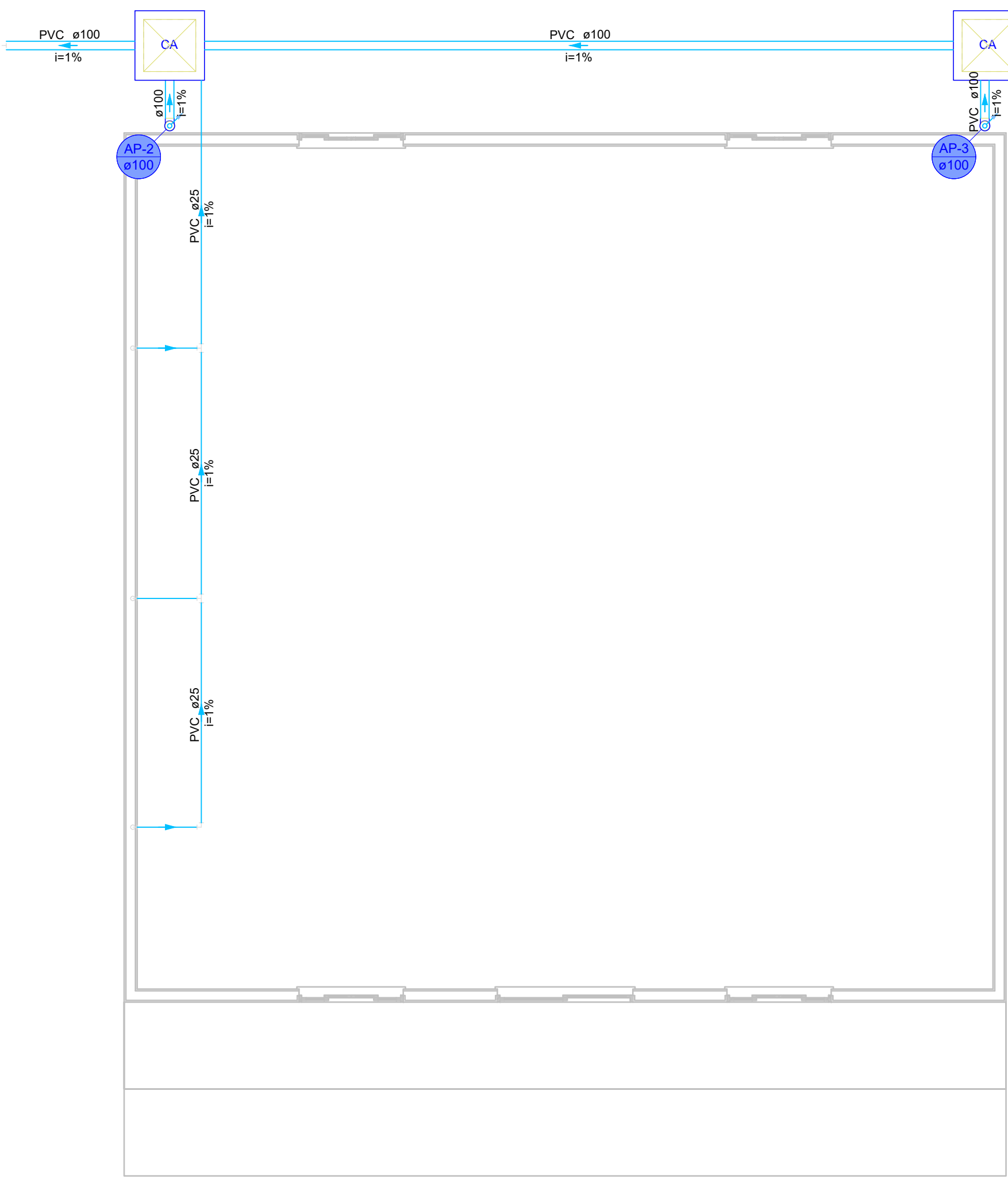
PLANTA BAIXA TÉRREO-SANITÁRIO ESC. 1/50
