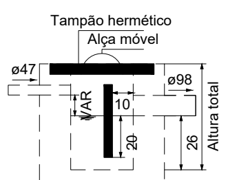
Caixa de gordura - TÉRREO
