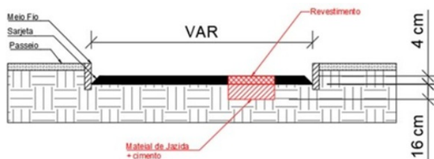
Figura 02 – Esquema de perfil transversal para reparo profundo.
