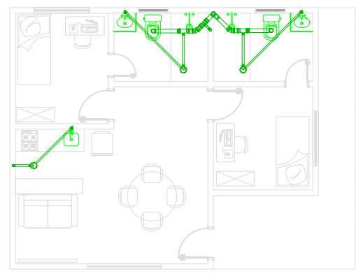
PLANTA ESGOTO MÓDULO ALOJAMENTO CONSTRUIDO SOBRE O MÓDULO ADMINISTRATIVO
