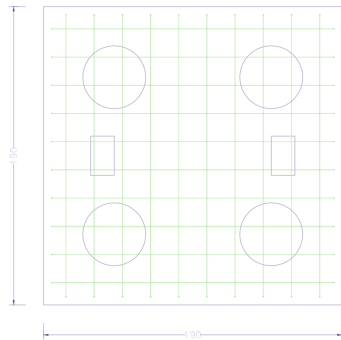
Estacas: D=40
