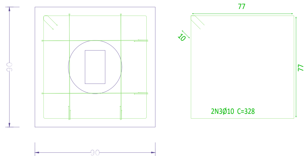
Estacas: D=40
