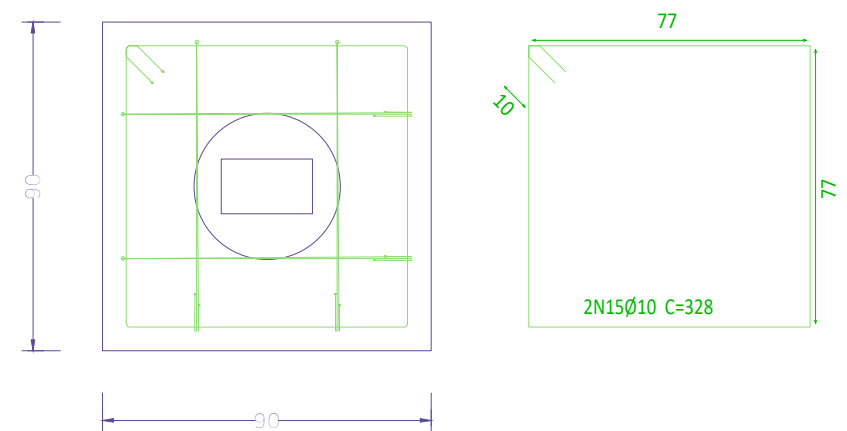
Estacas: D=40
