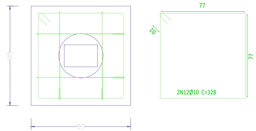
Estacas: D=40
