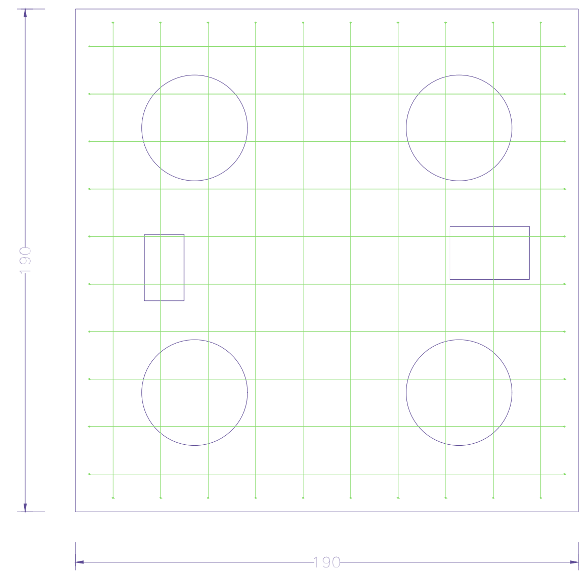
Estacas: D=40
