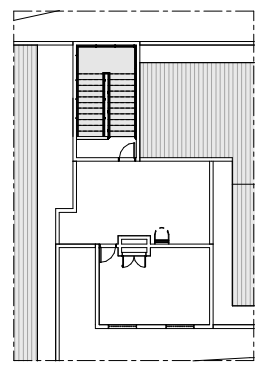
3 DETALHE PLANTA COBERTURA 1:75
