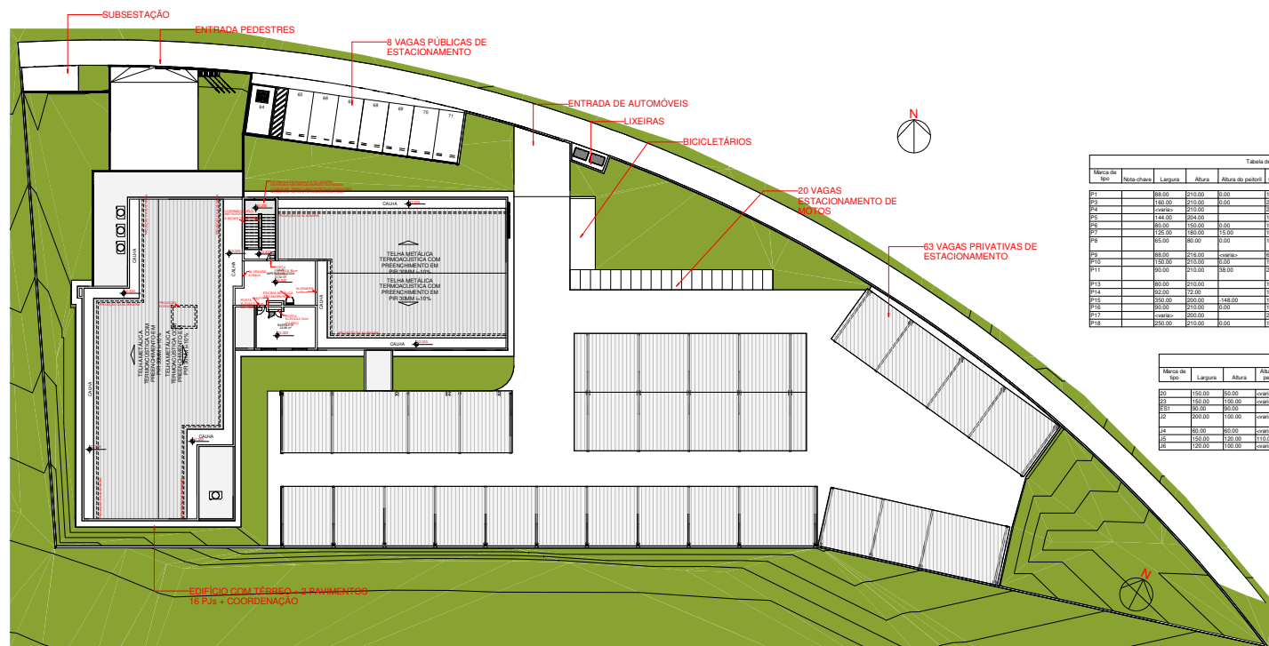
1 COBERTURA E IMPLANTAÇÃO 1:125
