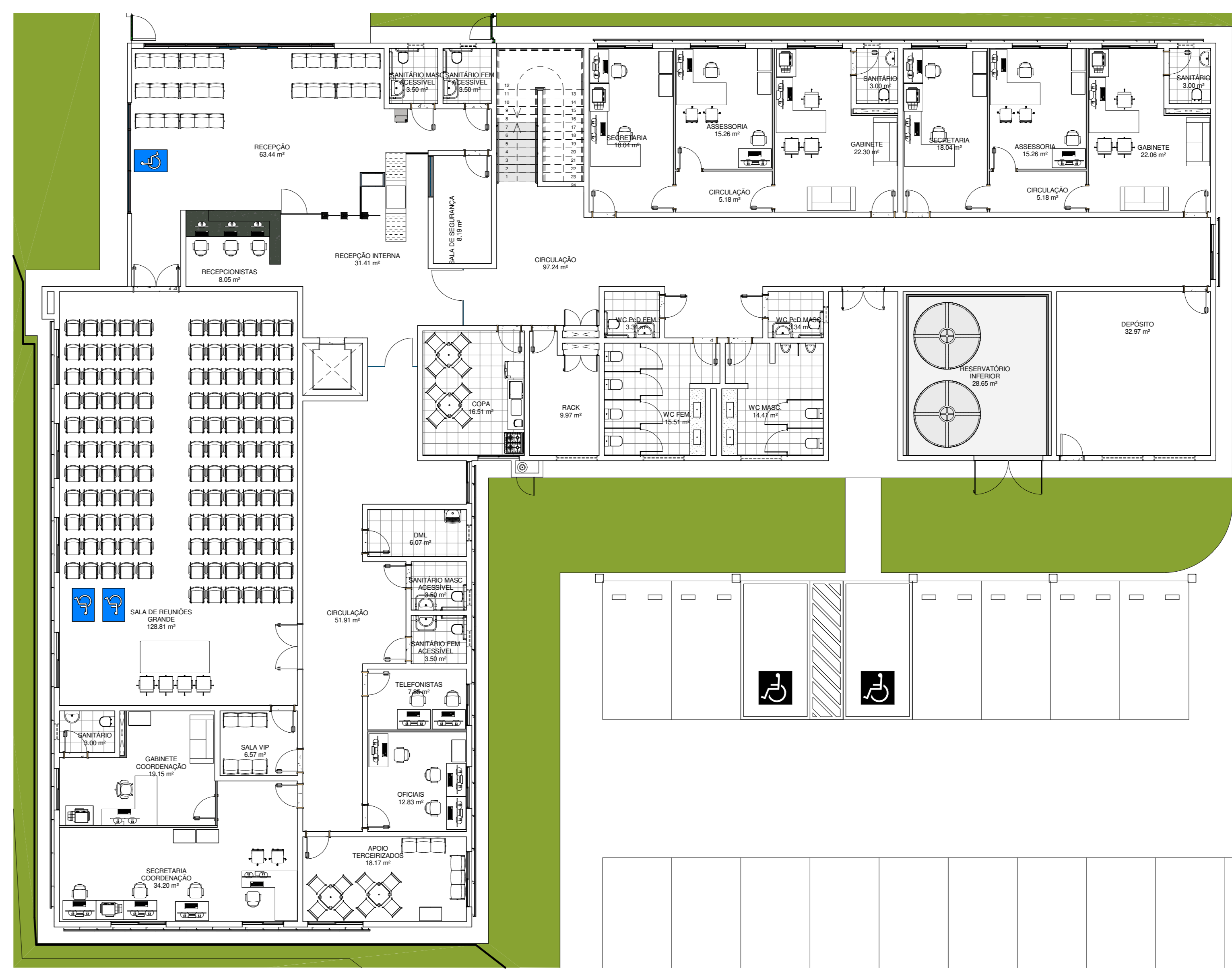
2 TÉRREO - LAYOUT 1:100
