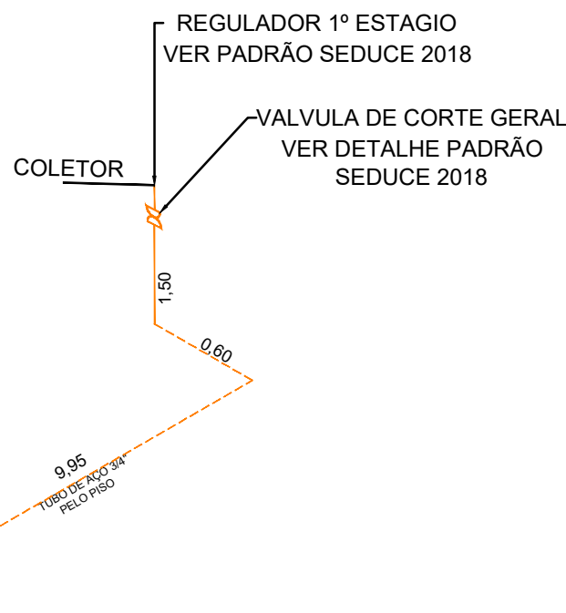
Planta baixa - Instalação de Gás Escala 1:100
