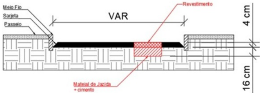
Figura 02 – Esquema de perfil transversal para reparo profundo.
