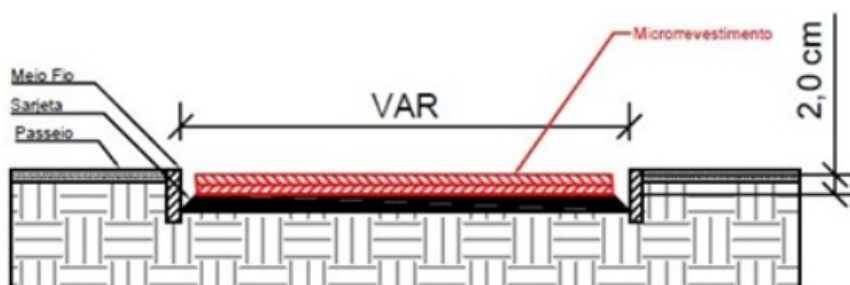
Figura 04 – Esquema de perfil transversal para Microrrevestimento.
