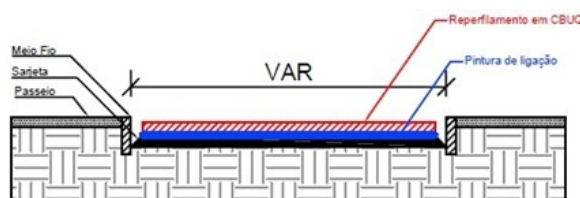
Figura 03 – Esquema de perfil transversal com destaque para pintura de ligação.
