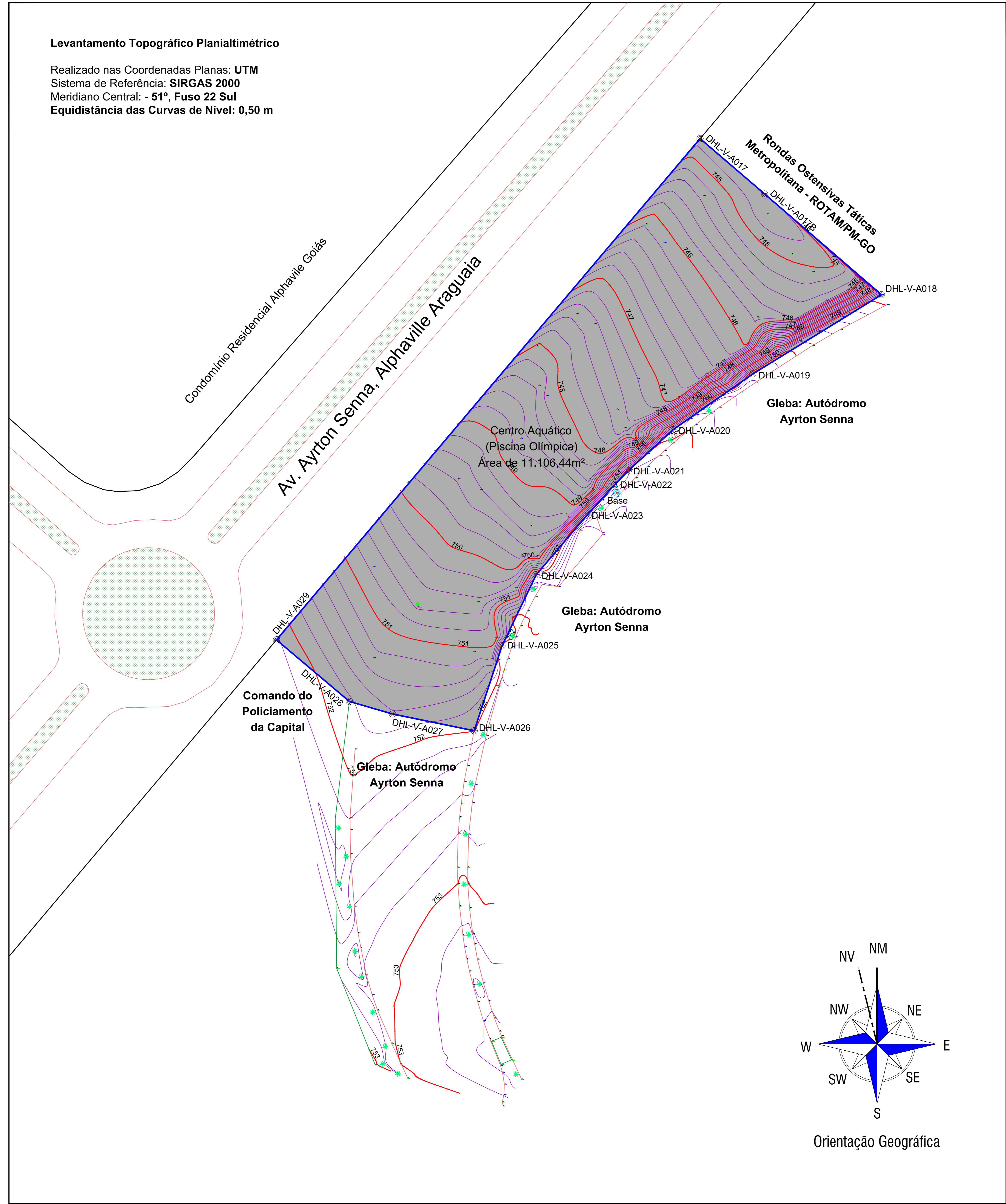
LEVANTAMENTO PLANIALTIMÉTRICO ESC.: 1/500
