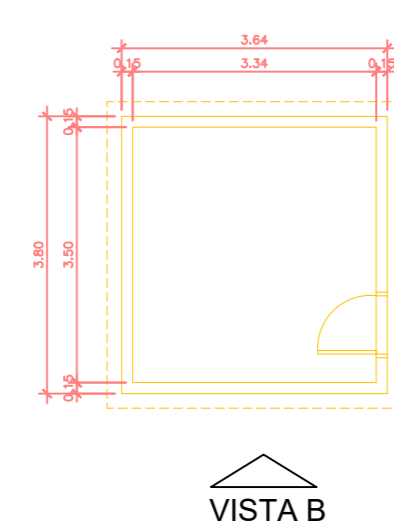
Planta baixa Casa de Bombas Escala 1:100
