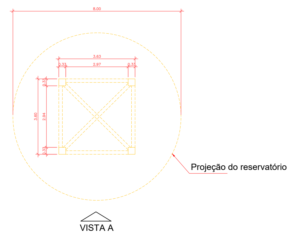
Planta baixa do reservatório Escala 1:100
