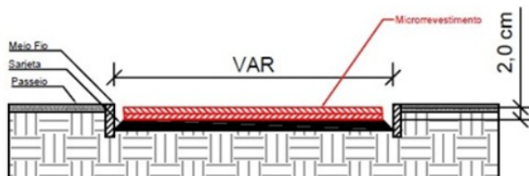
Figura 04 – Esquema de perfil transversal para Microrrevestimento.
