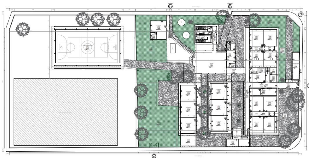
Imagem 02- Planta baixa da unidade.
