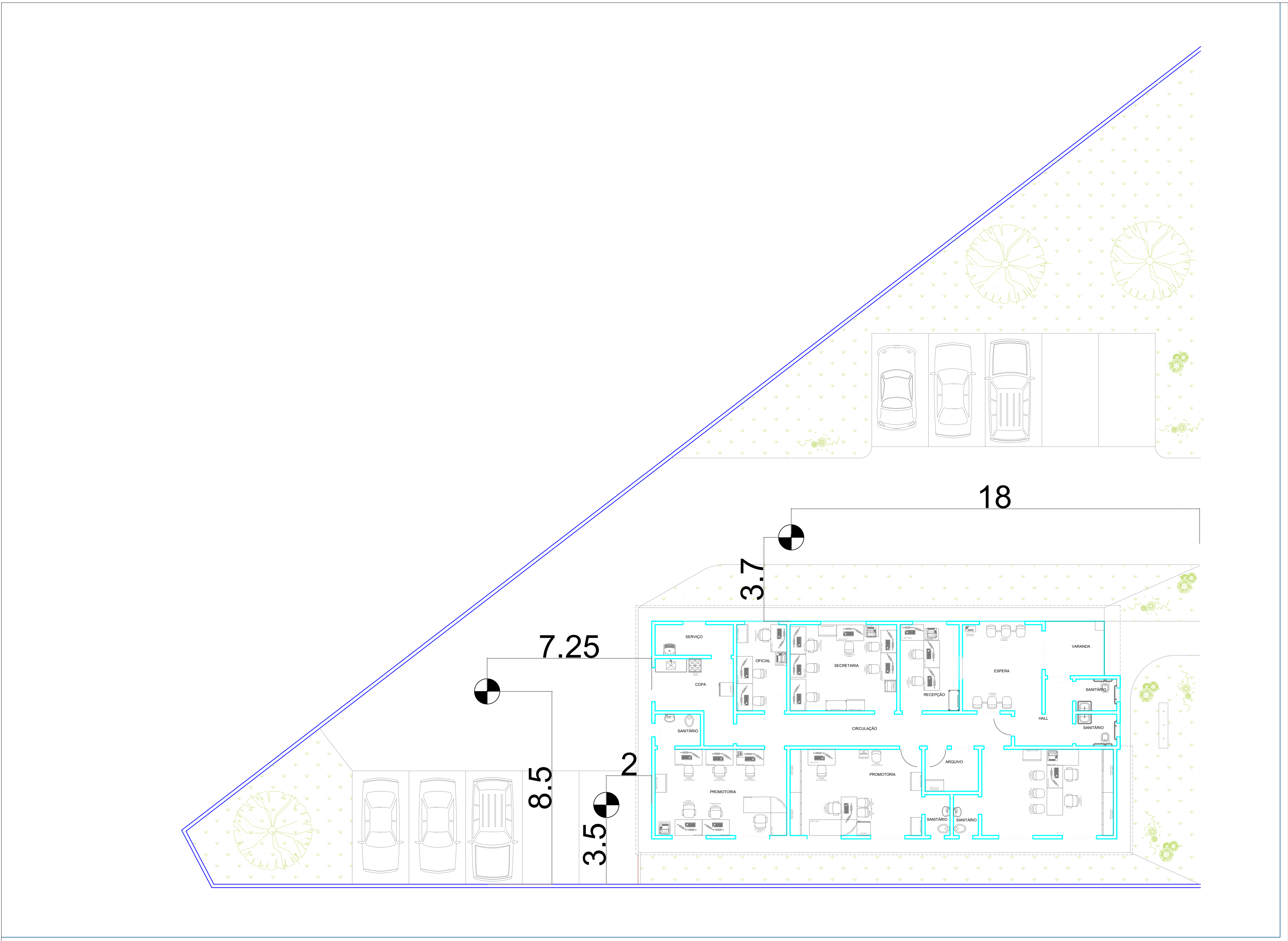
PLANTA MAPA DE LOCAÇÃO DE FUROS DE SONDAGEM ESC.: 1 : 250
