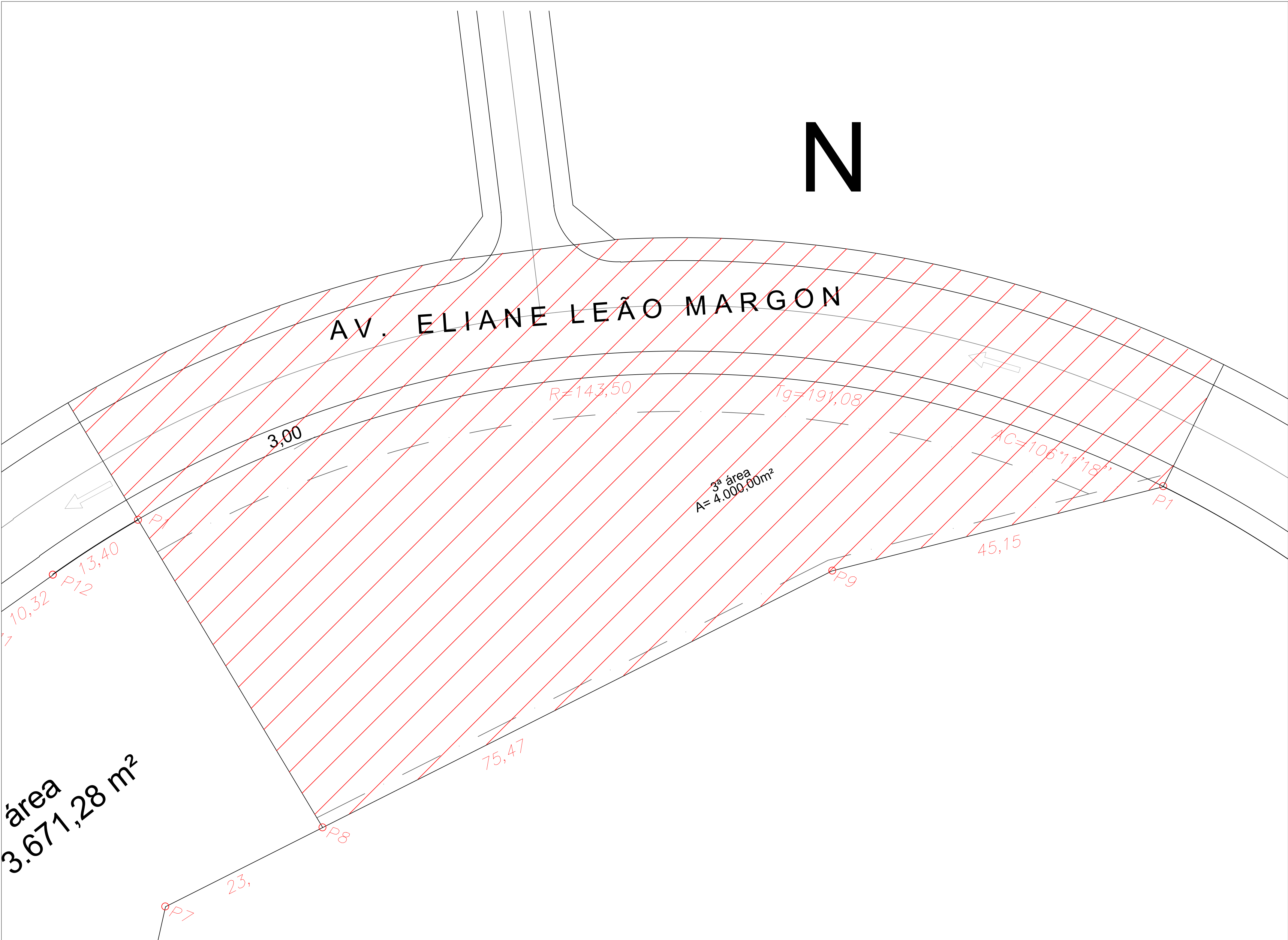
PLANTA MAPA PARA LEVANTAMENTO TOPOGRÁFICO ESC.: 1 : 300
