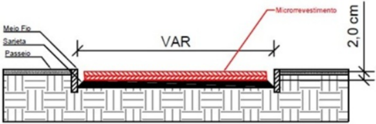
Figura 04 – Esquema de perfil transversal para Microrrevestimento.
