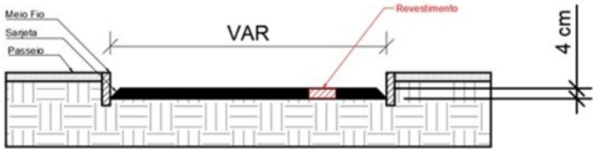
Figura 01 – Esquema de perfil transversal para reparo superficial.
