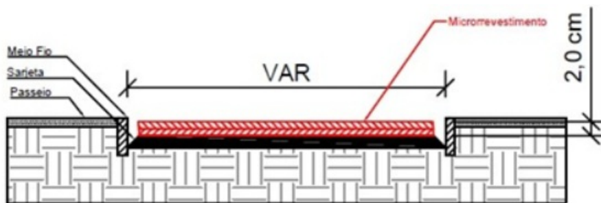
Figura 04 – Esquema de perfil transversal para Microrrevestimento.
