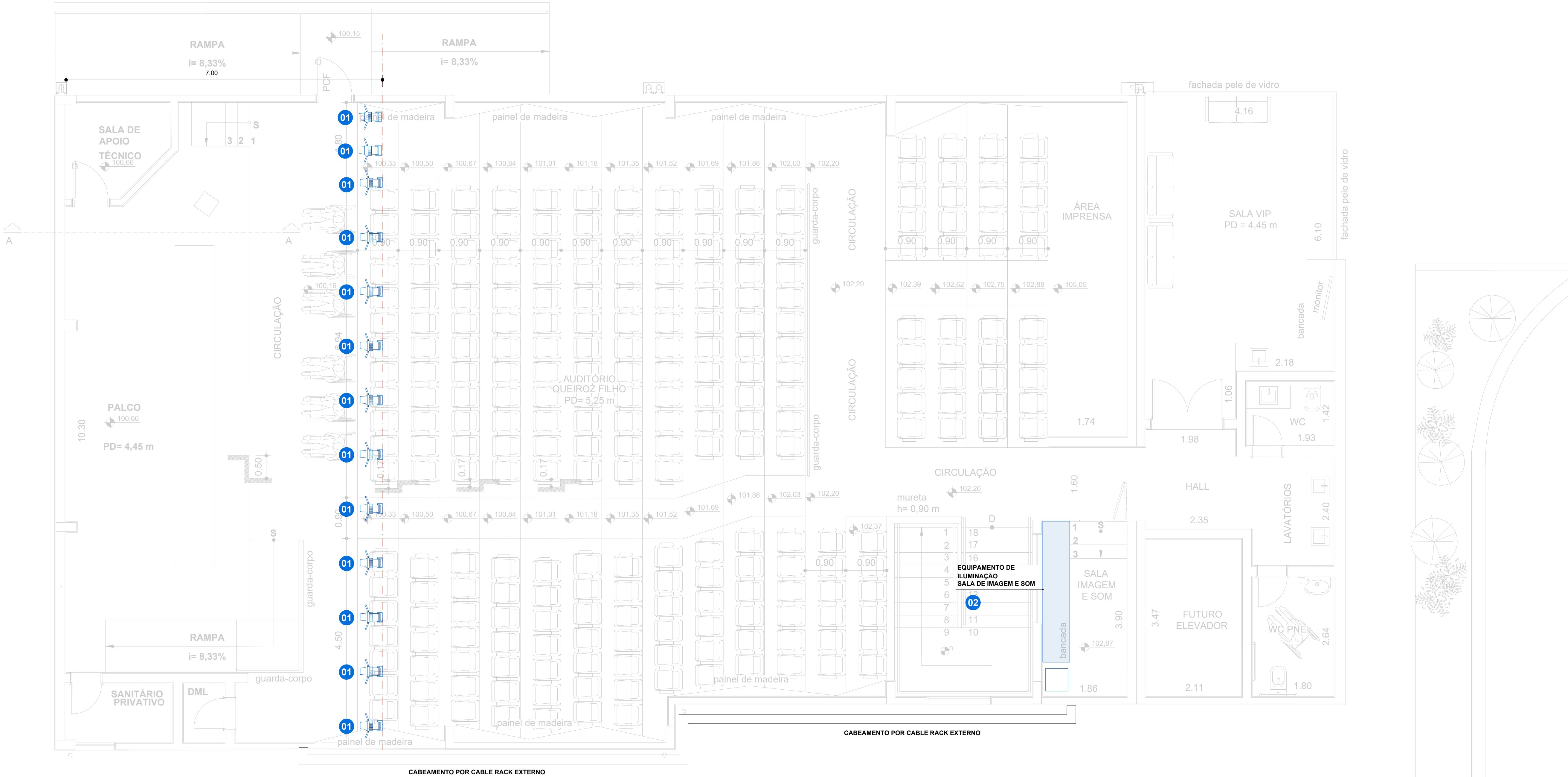
AUDITÓRIO QUEIROZ FILHO LAYOUT - SISTEMA DE ILUMINAÇÃO ESCALA 1:50
