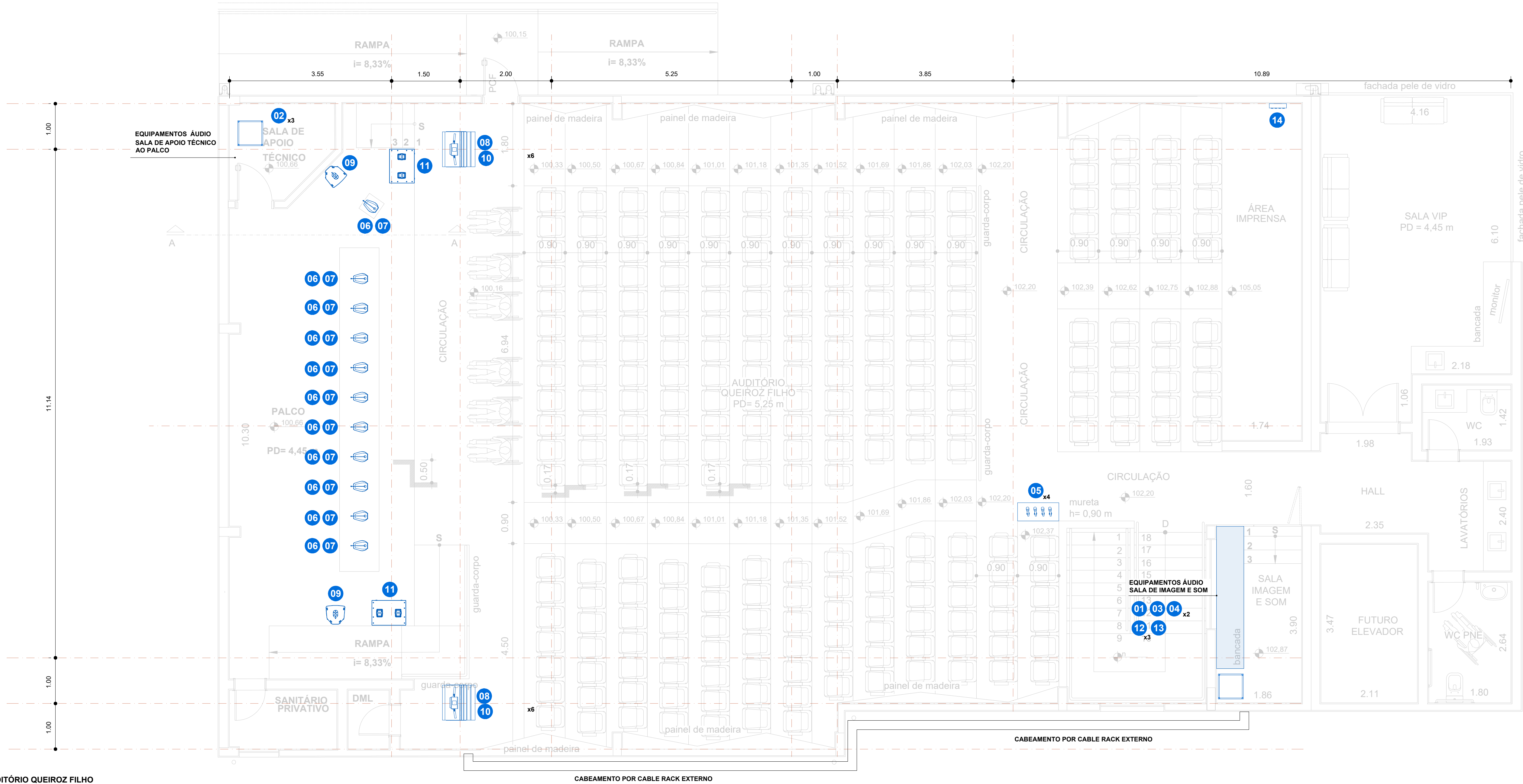
AUDITÓRIO QUEIROZ FILHO LAYOUT - SISTEMA DE ÁUDIO ESCALA 1:50
