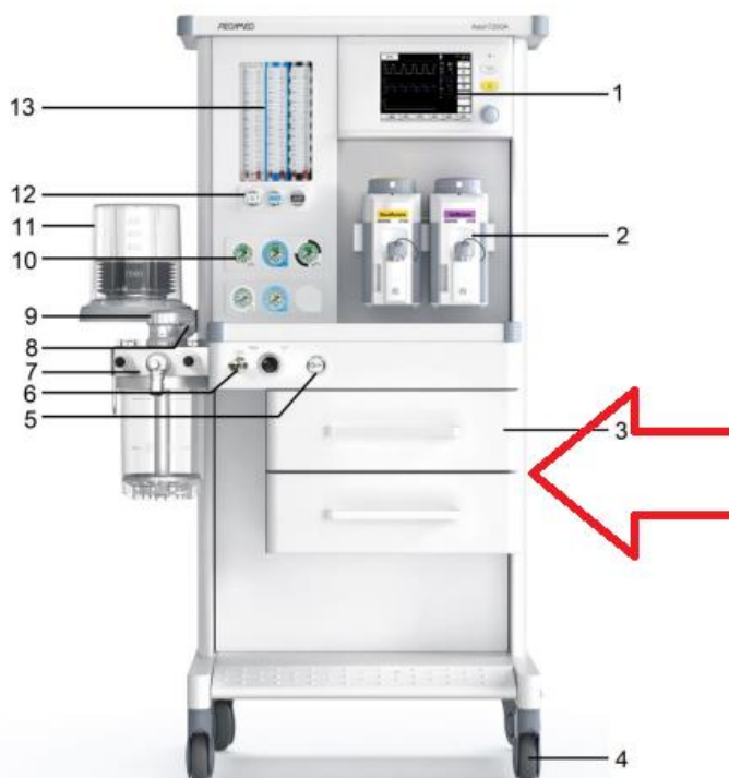
Figura 2-1 Vista Frontal
