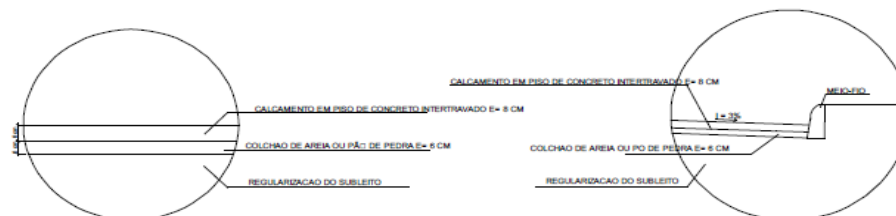
DETALHE - CAMADAS DE CALÇAMENTO Esc: Sem Escala
