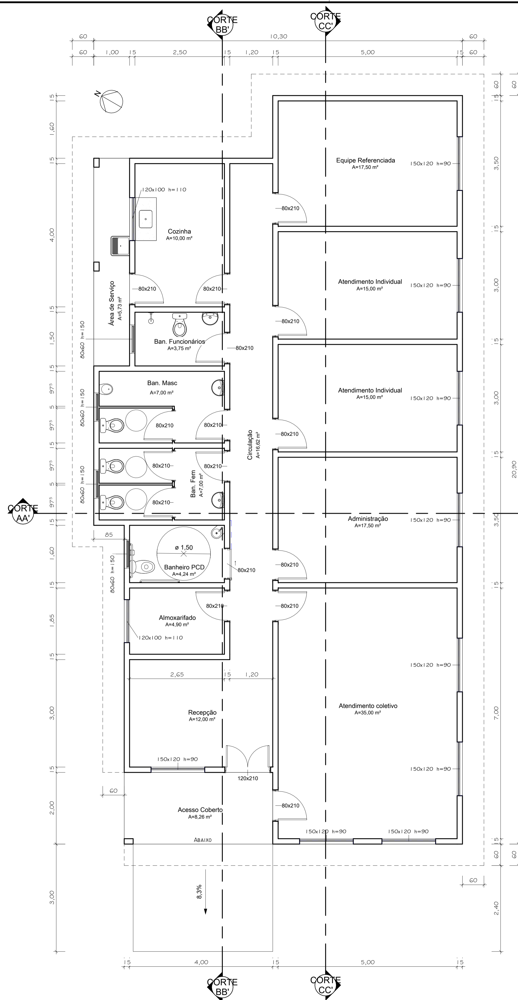
1 PLANTA BAIXA TÉRREO 1 : 50
