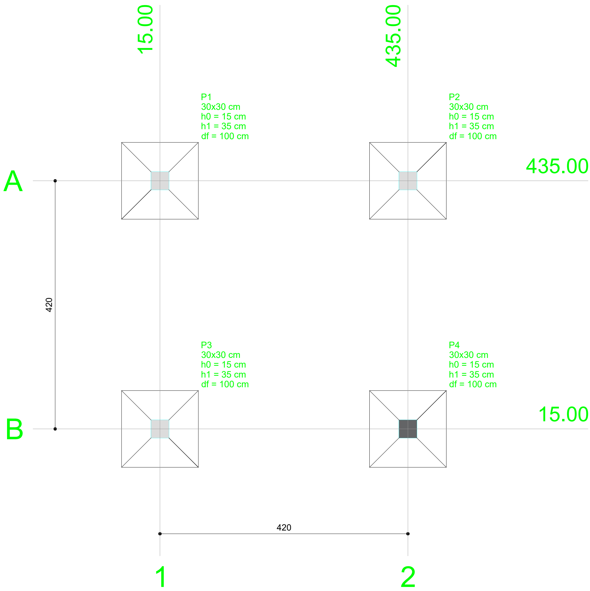
Planta de localização escala 1:50
