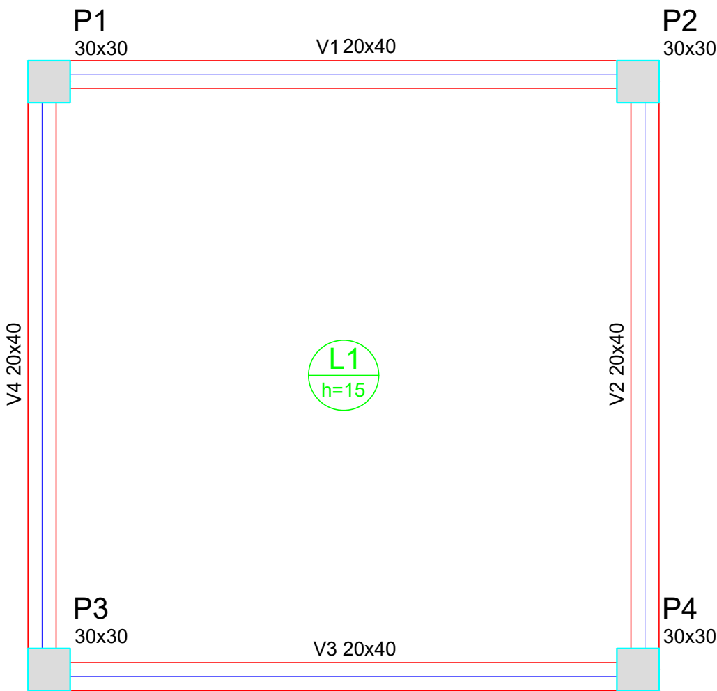
Forma do pavimento terreo escala 1:50
