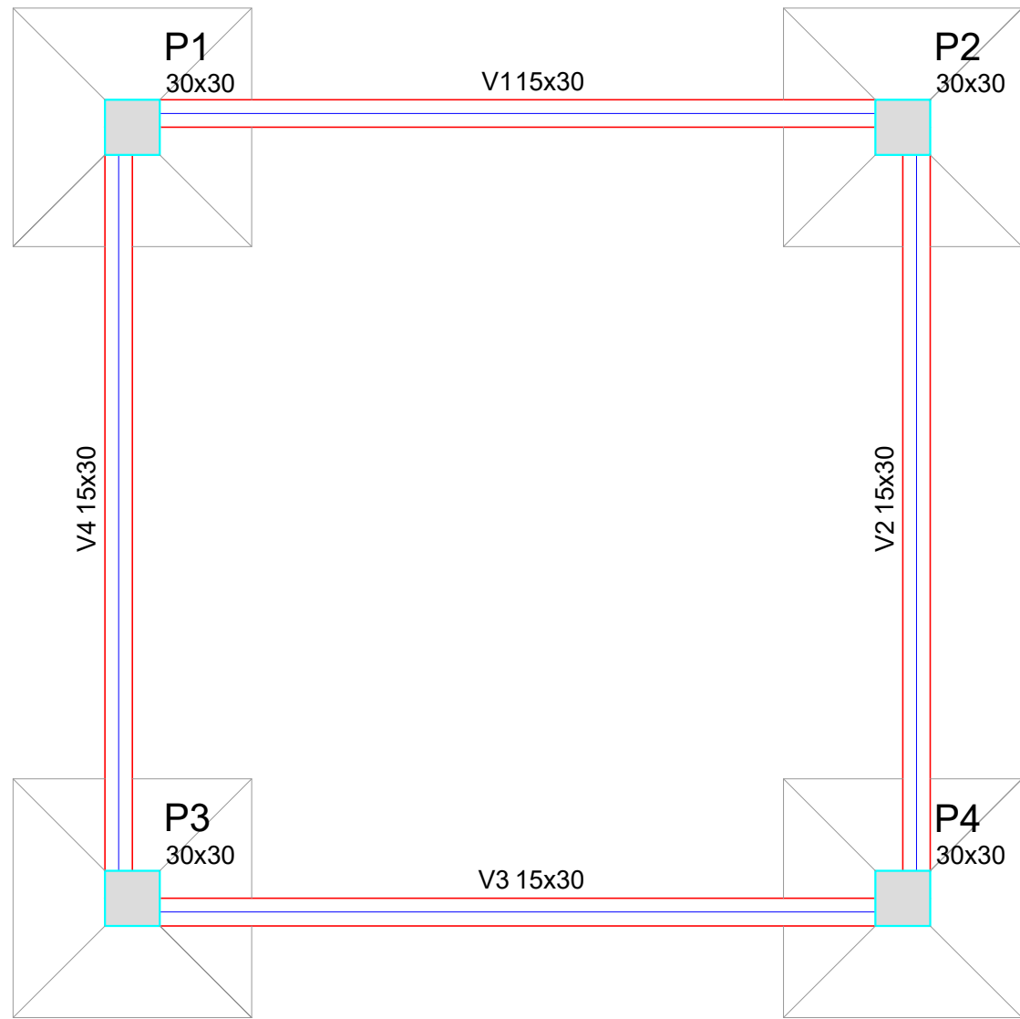
Forma do pavimento Fundação escala 1:50
